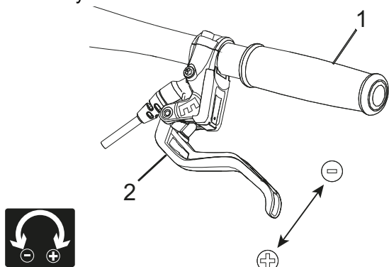
Illustration 49 : Régler la garde d'un levier de frein Magura HS33
