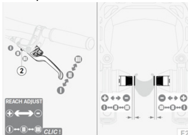
Illustration 50 : Régler la garde d'un levier de frein Magura HS22
