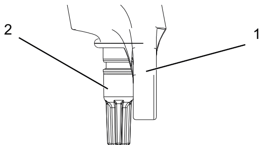
Rysunek 73: Nastawnik odbicia Suntour (2), widelec (1)
