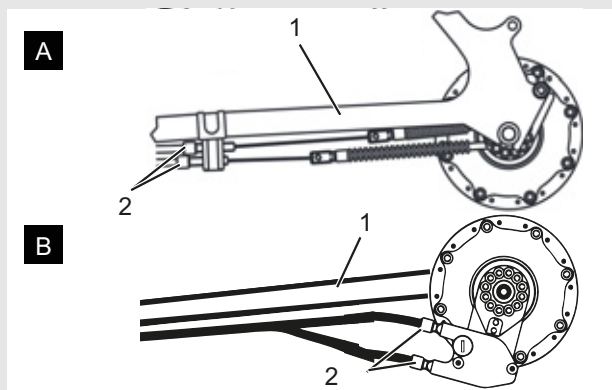
Rysunek 68: Nakrętki regulacyjne (2) w dwóch alternatywnych wersjach (A lub B) dwucięgnowego mechanizmu zmiany przerzutek na rurze dolnej tylnego trójkąta (1)
