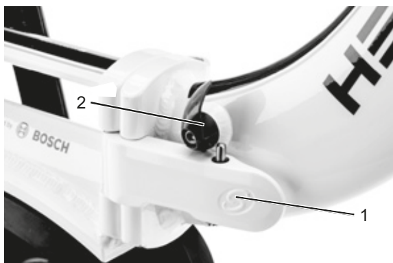
Afbeelding 73: Frame, met gesloten spanhendel (1) en geopende vergrendelhendel (2)
