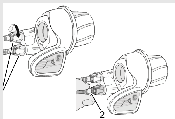
Afbeelding 99: Draaibare handvatschakelaar met afstelwartels (1) en speling van de versnelling (2)
