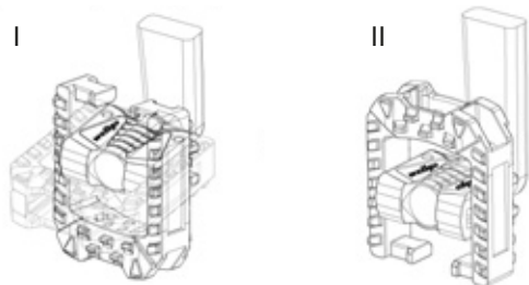
Afbeelding 70: Pedaal omlaag (I) of omhoog (II) invouwen
