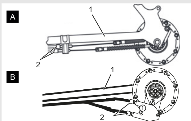
Afbeelding 98: Afstelwartels (2) van twee alternatieve uitvoeringen (A resp. B) van een versnelling met dubbele bowdenkabelbediening aan de achterbrug (1)
