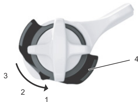
Afbeelding 86: Fijnafstelling van de stand OPEN met de afsteller (4)
