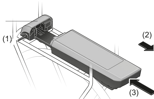
Afbeelding 78: Bagagedrageraccu verwijderen (2) en aanbrengen (3)
