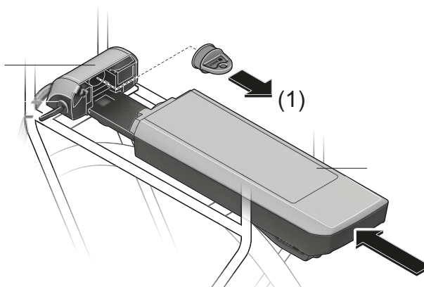
Afbeelding 81: Open contacten afdekken met afdekkap, voorbeeld bagagedrageraccu
