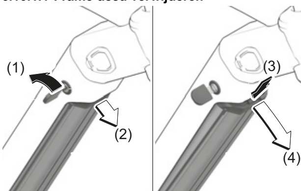
Afbeelding 77: Frame-accu verwijderen en aanbrengen
