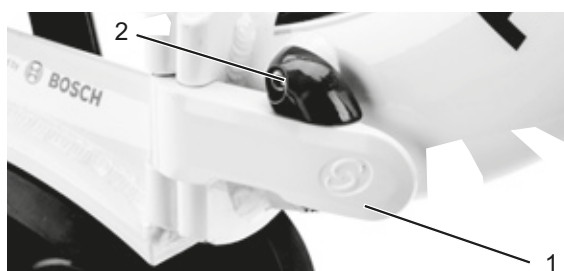
Afbeelding 74: Frame, met gesloten spanhendel (1) en gesloten vergrendelhendel (2) van het frame. Pedaal uitvouwen
