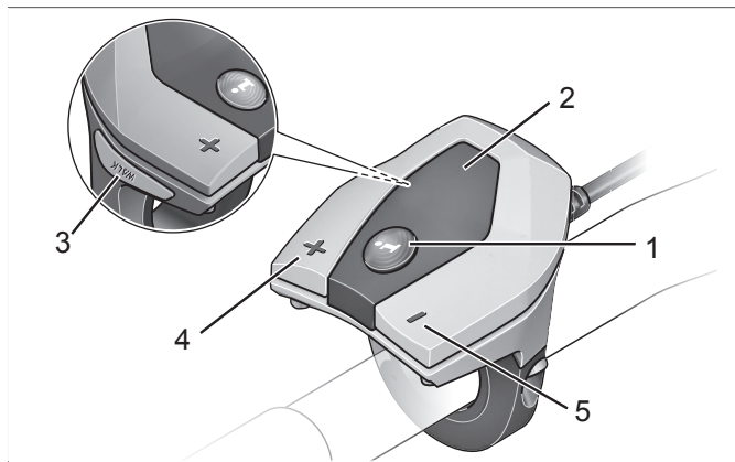
Übersicht Bedienteil
