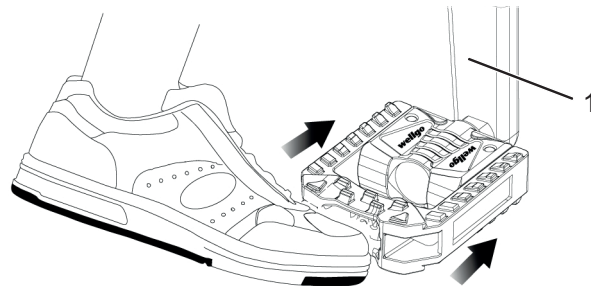
Abbildung 42: Pedal gegen Tretkurbel (1) drücken
