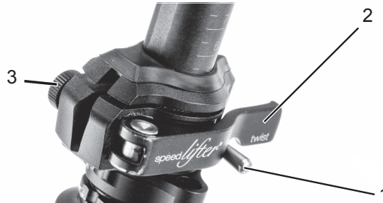
Abbildung 23: Geschlossener Spannhebel (2) mit Rändelmutter (3) und Sicherungshebel (1) am Vorbau
