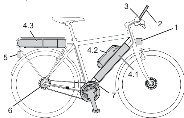
Figura 6: Schema del sistema di trazione elettrica
