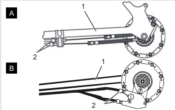
Figura 41: Boccole di regolazione (2) di due versioni alternative (A e B) di un cambio azionato da cavo doppio sul fodero orizzontale (1)
