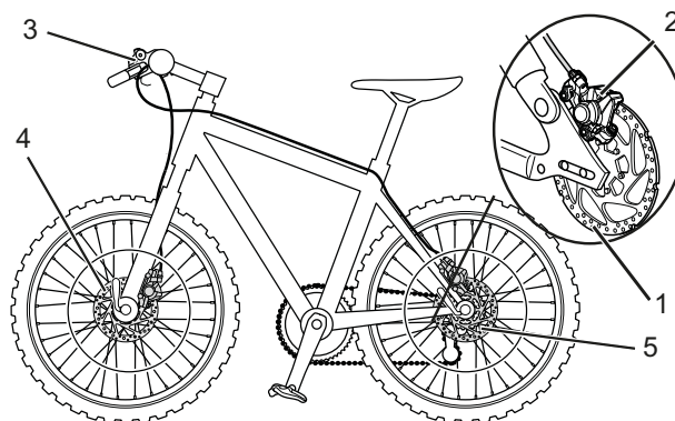
Figura 4: Sistema frenante con freno a disco, esempio
