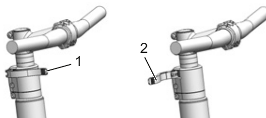
Figura 26: Leva di serraggio dell'attacco manubrio chiusa (1) e aperta (2), esempio All Up
