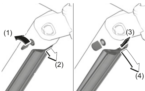
Figura 31: Smontaggio della batteria integrata
