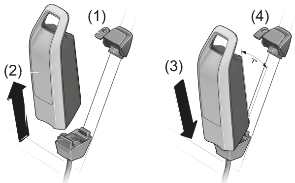
Figura 29: Smontaggio e montaggio della batteria sul tubo trasversale
