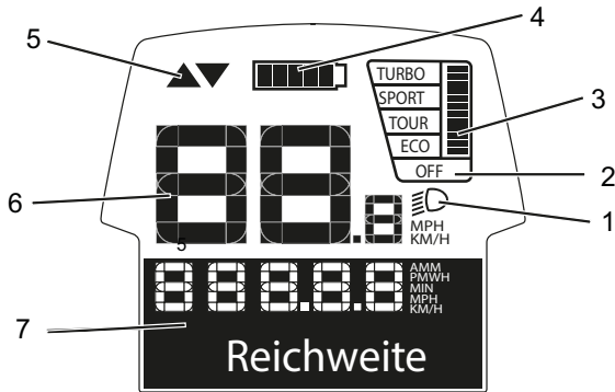
Figura 18: Schema degli indicatori sul display
