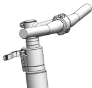
Rysunek 139: Kierownica typu All Up z otwartą dźwignią mocującą mostek
