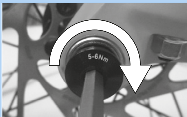
Rysunek 65: Sposób dokręcania śruby zabezpieczającej
