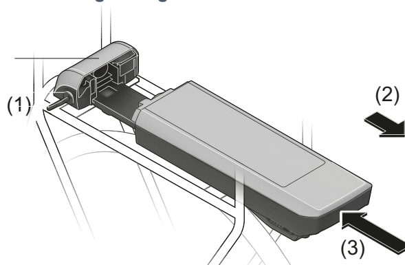
Rysunek 121: Wymywanie (2) i wkładanie (3) akumulatora zintegrowanego z bagażnikiem
