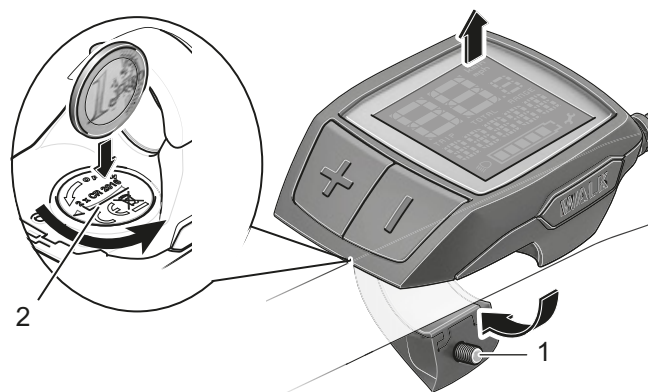
Rysunek 126: Komputer pokładowy ze śrubą mocującą (1) i pokrywą komory baterii (2)
