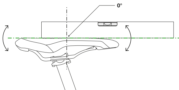
Rysunek 87: Poziome ustawienie siodełka z nachyleniem 0° jego środkowej części
