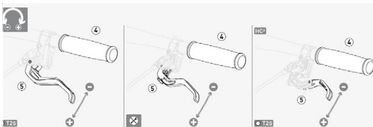
Rysunek 103: Ustawianie odchylenia manetki dźwigni hamulca tarczowego MAGURA
