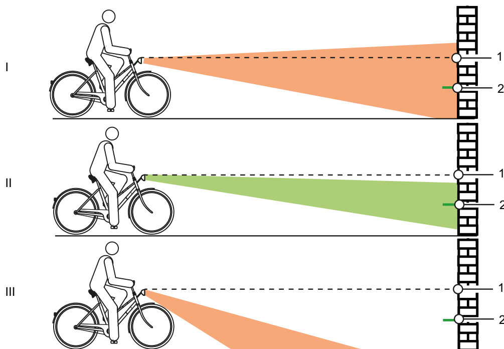
Rysunek 149: Światło ustawione za wysoko (1), prawidłowo (2) i za nisko (3)
