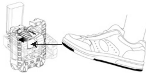
Rysunek 137: Dociskanie pedału do korby (1)
