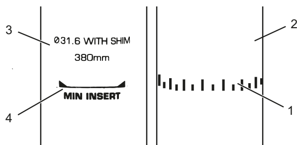
Rysunek 84: Widok szczegółowy sztycy podsiodłowych, przykłady oznaczenia minimalnej głębokości osadzenia
