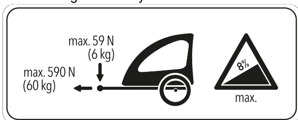
Rysunek 113: Tabliczka informacyjna przyczepki
