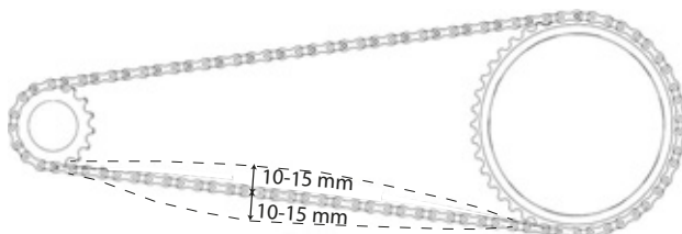
Rysunek 150: Kontrola naprężenia łańcucha
