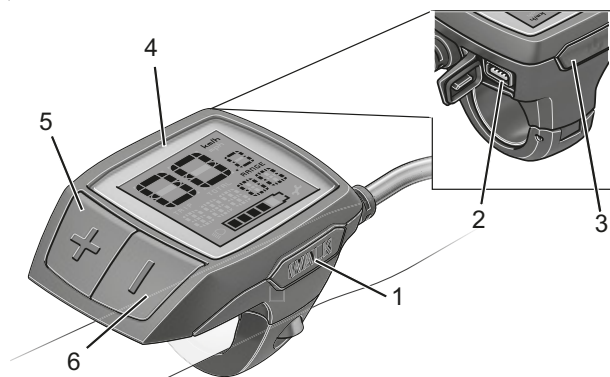
Rysunek 112: Budowa komputera pokładowego Purion firmy BOSCH
