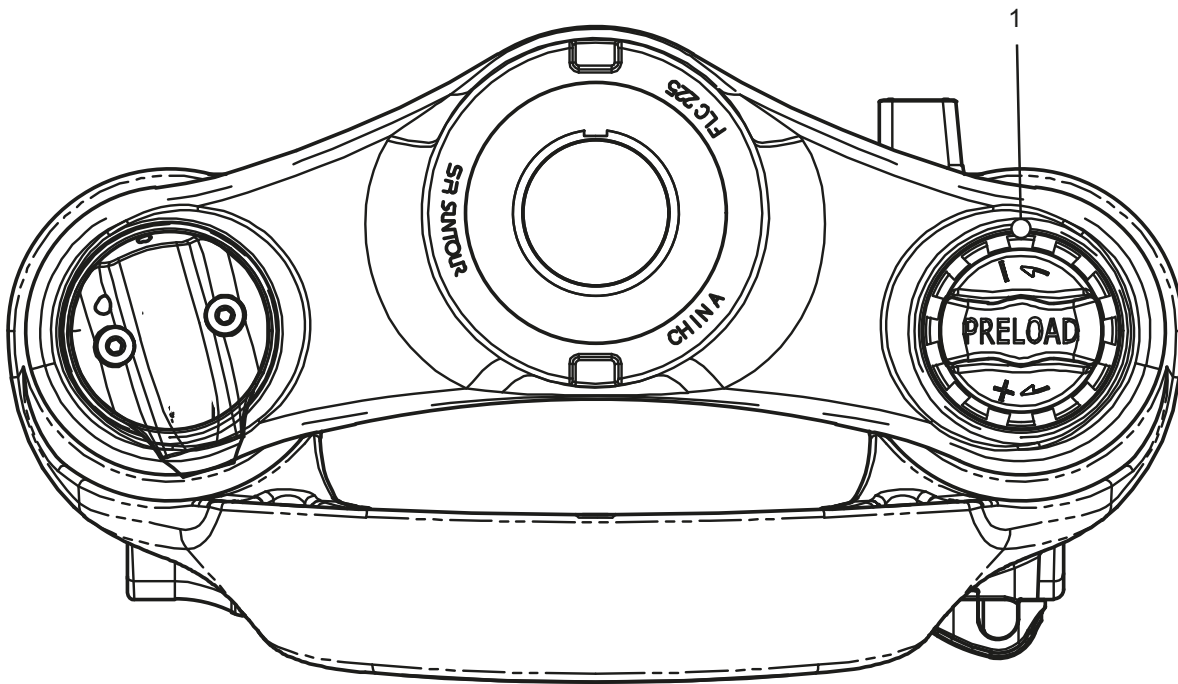
Rysunek 105: Pokrętko regulacyjne parametru SAG (1) usytuowane na koronie widelca amortyzowanego
