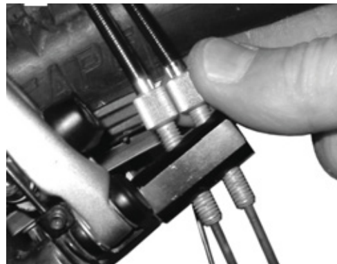
Rysunek 151: Wersje piast Rohloff z wewnętrznym sterowaniem zmiany biegów posiadają regulator naprężenia na wsporniku linek
