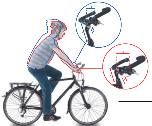
Rysunek 95: Pozycja roweru miejskiego (niebieski) i trekkingowego (czerwony) dzięki regulacji kąta nachylenia
