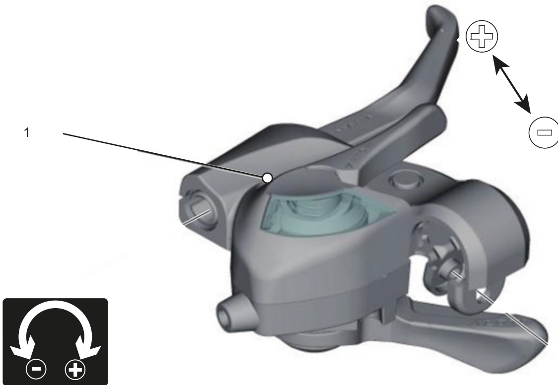
Rysunek 104: Pozycja śruby regulacyjnej (1)
