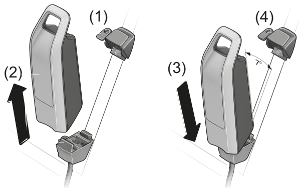
Rysunek 120: Wymywanie i wkładanie akumulatora zintegrowanego z ramą
