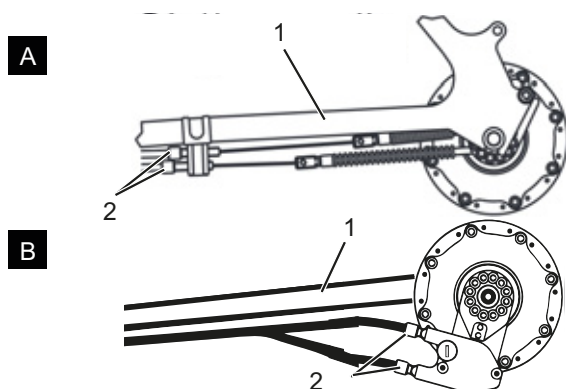
Rysunek 154: Nakrętki regulacyjne (2) w dwóch alternatywnych wersjach (A i B) dwucięgowego mechanizmu zmiany przerzutek na rurze dolnej tylnego trójkąta (1)
