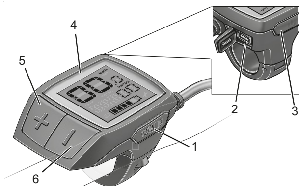
Rysunek 37: Budowa komputera pokładowego Purion firmy BOSCH
