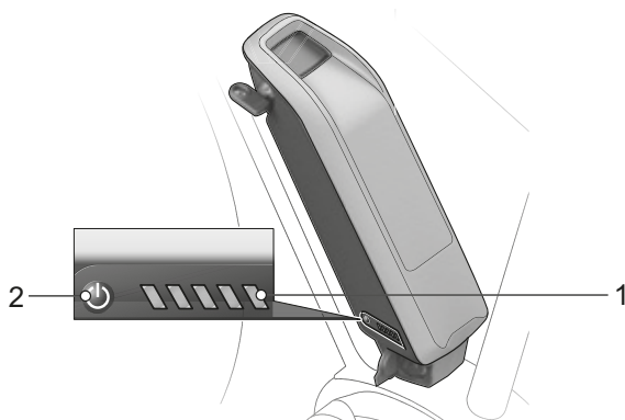
Rysunek 43: Pozycja wskaźnika stanu naładowania na akumulatorze na rurze podsiodłowej
