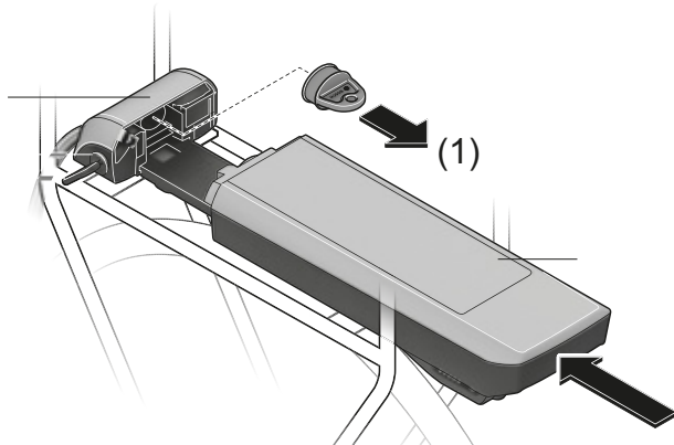
Rysunek 124: Zasłonić odsłonięte styki osłoną, przykład – bagażnik
