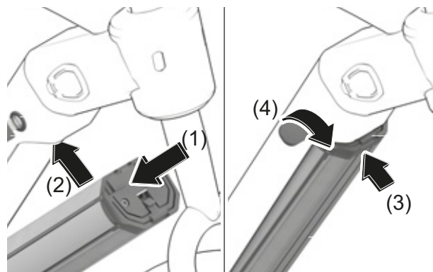
Rysunek 123: Wkładanie zintegrowanego akumulatora
