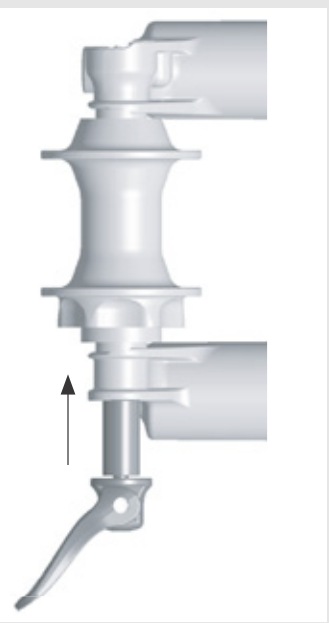
Figura 41: Inseririmento del bloccaggio rapido
