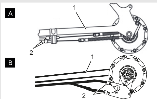
Rysunek 76: Nakrętki regulacyjne (2) w dwóch alternatywnych wersjach (A lub B) dwuczęściowego mechanizmu zmiany przerzutek na rurze dolnej tylnego trójkąta (1)
