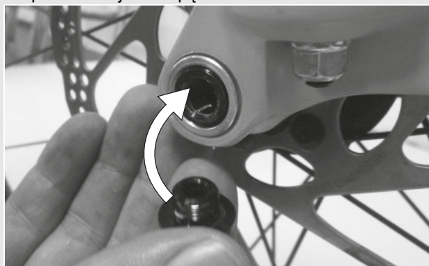
Rysunek 22: Sposób wsuwania dźwigni zacisku szybko mocującego w oś
