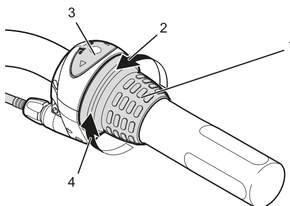
Rysunek 71: Przykładowy mechanizm zmiany przerutek marki Shimano Nexus: Manetka obrotowa (1) przekładni w piąście ze wskaźnikiem (3), kierunek obrotu przy zmianie na wyższy bieg (2) i na niższy bieg (4)
