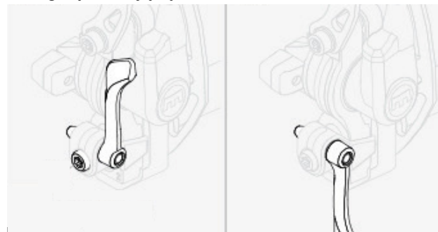
Rysunek 10: Dźwignia blokująca hamulec obręczowy na kole zamknięta (1) i otwarta (2)
