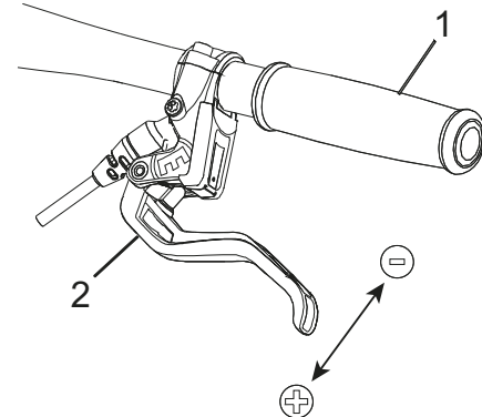
Rysunek 51: Ustawianie odległości dźwigni hamulca od uchwytu kierownicy (1) za pomocą śruby regulacyjnej (2)
