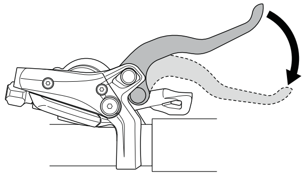
Rysunek 50: Odchylenie manetki dźwigni hamulca
