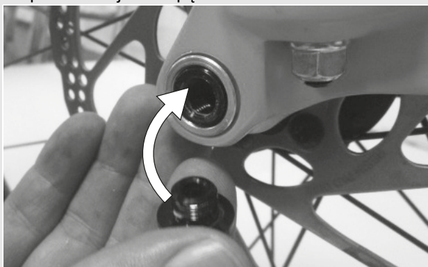
Rysunek 27: Sposób wsuwania dźwigni zacisku szybko mocującego w oś
