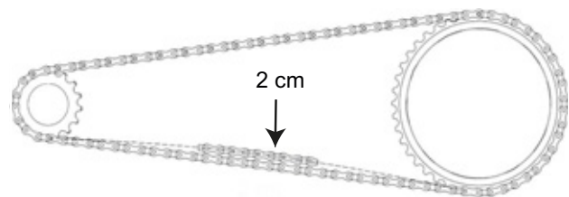
Rysunek 83: Kontrola naprężenia łańcucha
