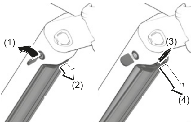
Rysunek 68: Wymywanie wbudowanego akumulatora
