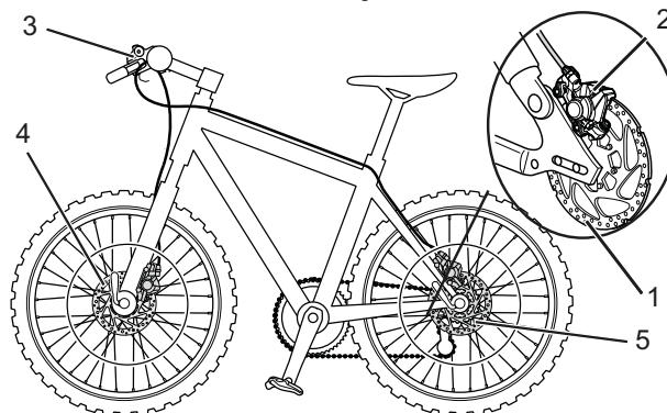
Rysunek 4: Układ hamulcowy wyposażony w hamulec tarczowy – przykład
