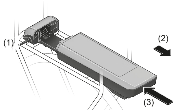
Rysunek 30: Wymywanie (2) i wkładanie (3) akumulatora zintegrowanego z bagażnikiem
