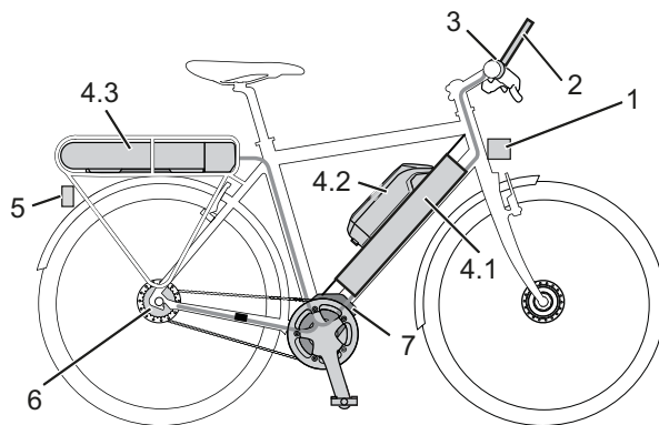
Rysunek 6: Schemat elektrycznego układu napędowego
