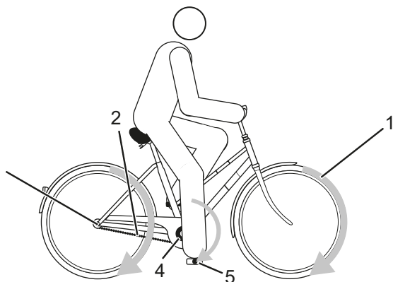
Rysunek 5: Schemat mechanicznego układu napędowego
