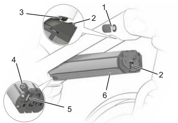
Rysunek 11: Szczegóły zintegrowanego akumulatora
