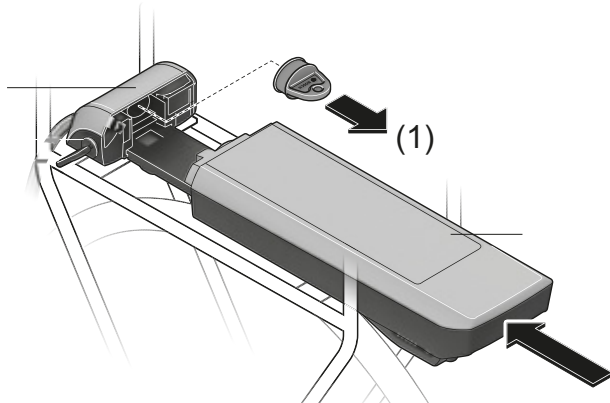
Rysunek 33: Zasłonić odsłonięte styki osłoną, przykład – bagażnik
