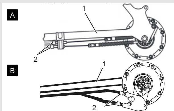
Rysunek 41: Nakrętki regulacyjne (2) w dwóch alternatywnych wersjach (A lub B) dwucięgnowego mechanizmu zmiany przerzutek na rurze dolnej tylnego trójkąta (1)
