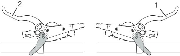
Rysunek 35: Dźwignia hamulca tylna (1) i przednia (2), przykład – hamulec Shimano
