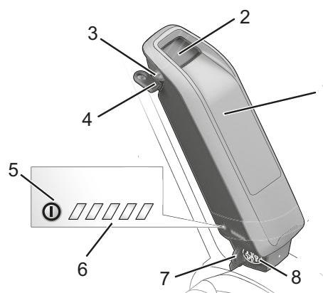
Rysunek 7: Szczegóły akumulatora zintegrowanego z ramą
