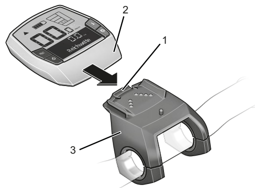
Rysunek 34: Wsunąć ekran (2) przez blokadę ekranu (1) do oporu w uchwyt (3)
