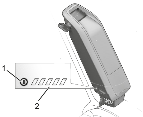
Figura 15: Indicador de carga en el ejemplo de la batería en el cuadro
