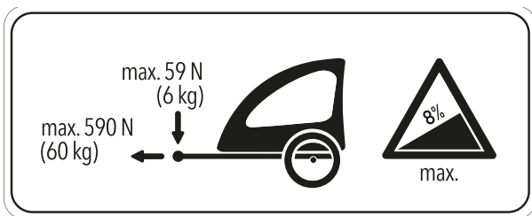
Figura 28: Placa indicadora de remolque
