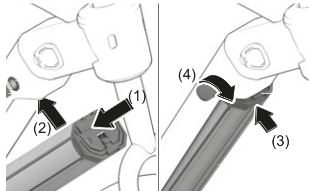
Figura 32: Inserción de la batería integrada
