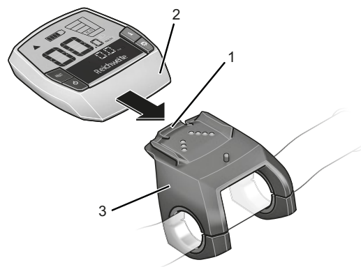
Figura 34: Inserción de la pantalla (2) a través del tope móvil de la pantalla (1) hasta el tope del soporte (3)
