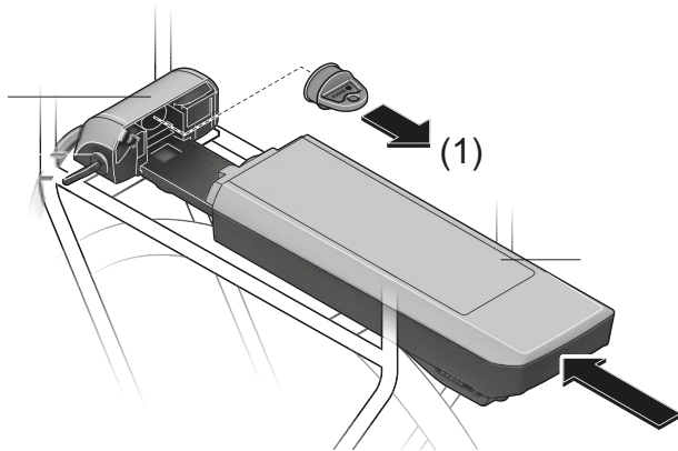
Figura 33: Cierre de los contactos abiertos con tapa de cierre, ejemplo batería del portaequipajes
