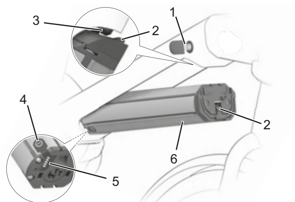
Figura 11: Detalle de la batería integrada
