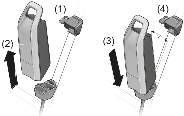
Figura 29: Extracción e inserción de la batería en el cuadro
