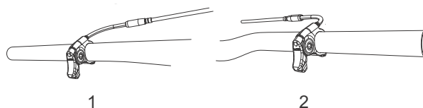
Figura 24: Palanca de la tija de sillín montada a la izquierda (1) o la derecha (2) del manillar.
