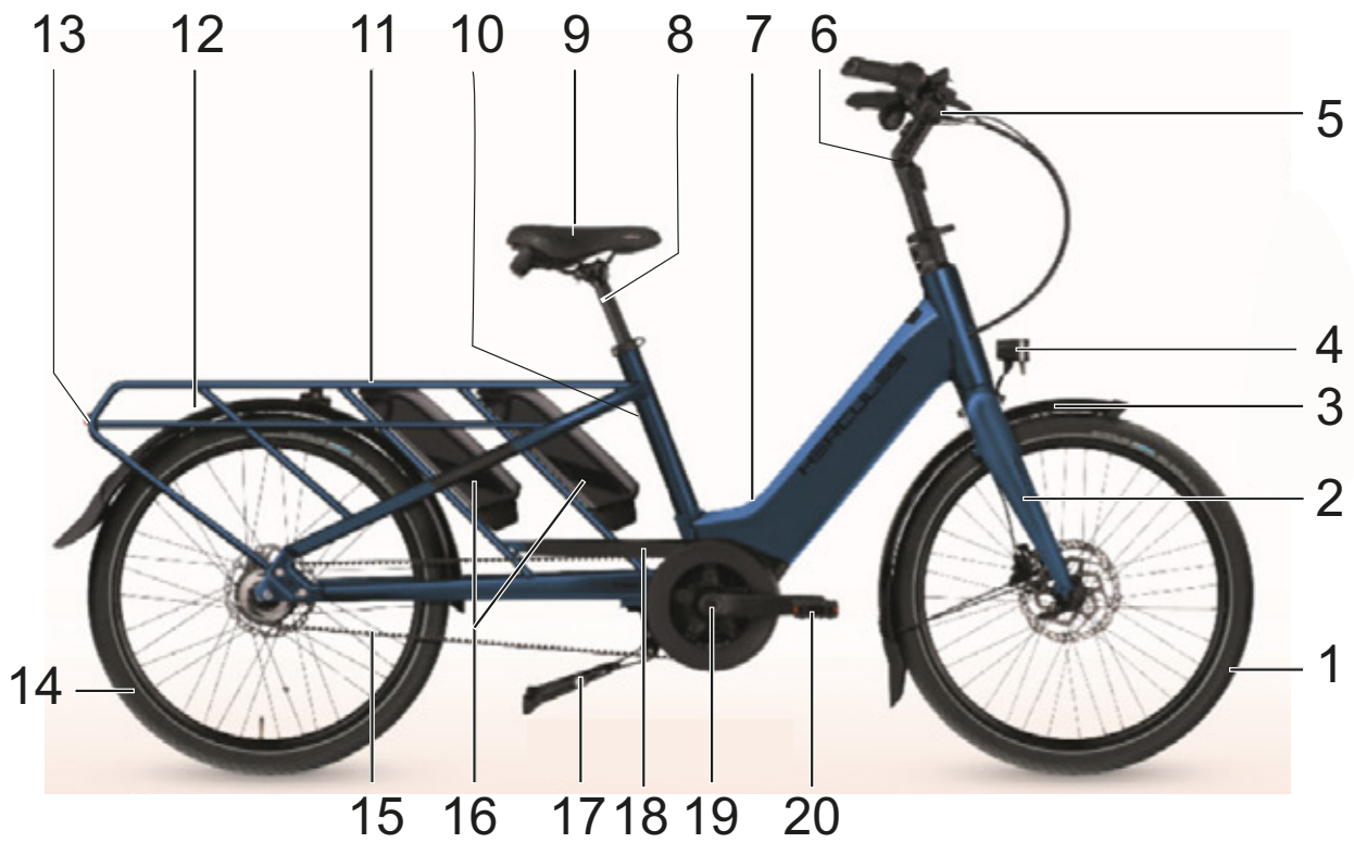
Figura 2: Pedelec visto desde el lado derecho, HERCULES Rob Family F360
