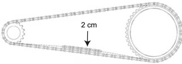
Figura 37: Comprobación de la tensión de la cadena
