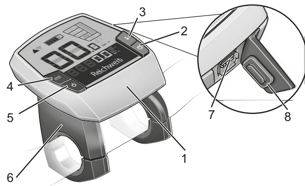
Figura 16: Vista general de la estructura y los elementos de mando de la pantalla
