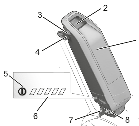
Figura 7: Detalle de la batería en el cuadro
