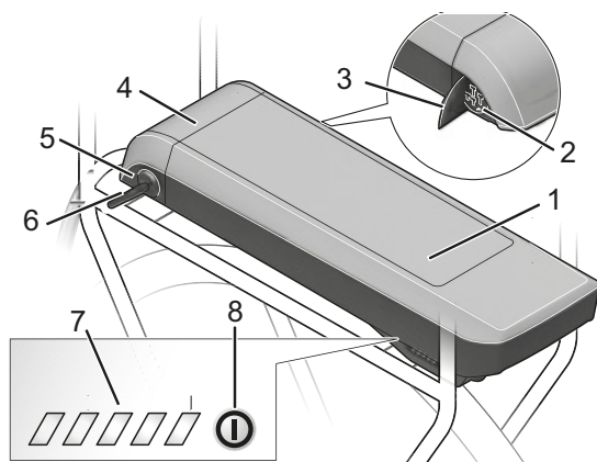
Figura 9: Detalle de la batería del portaequipajes
