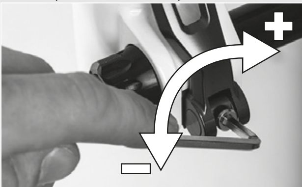
Figura 39: Ajuste de la fuerza de tensado del cierre rápido
