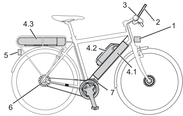
Figura 6: Esquema del sistema de accionamiento eléctrico
