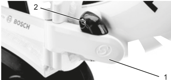
Rysunek 74: Rama z zamkniętą dźwignią mocującą (1) i zamkniętą dźwignią zabezpieczającą (2), rozłożyć pedały
