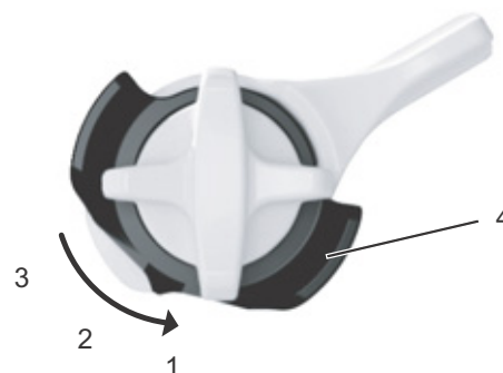
Rysunek 86: Do precyzyjnego ustawiania pozycji OTWARTE służy nastawnik (4)
