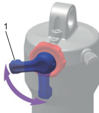
Rysunek 91: Ustawianie twardości tłumika dobicia za pomocą dźwigni (1) tylnego amortyzatora
