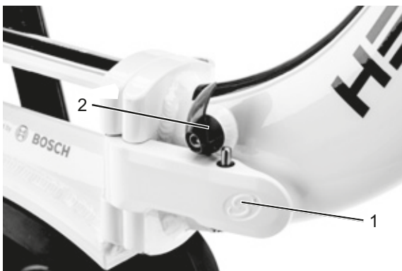
Rysunek 73: Rama z zamkniętą dźwignią mocującą (1) i otwartą dźwignią zabezpieczającą (2)
