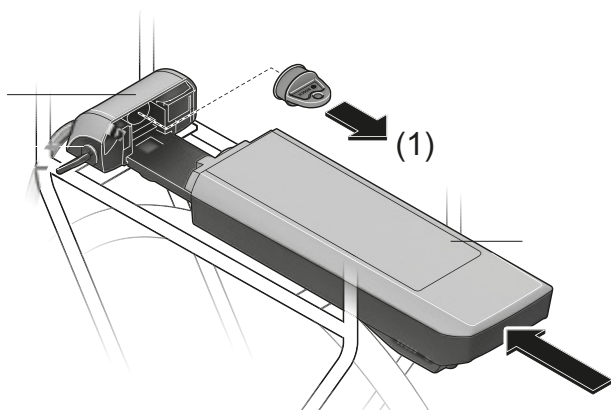
Rysunek 81: Zasłonić odsłonięte styki osłoną, przykład – bagażnik
