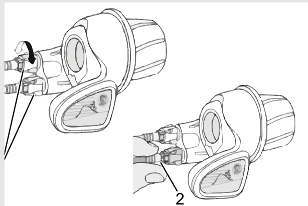
Rysunek 99: Manetka obrotowa z nakrętkami regulacyjnymi (1) i luzem mechanizmu zmiany przerzutek (2)
