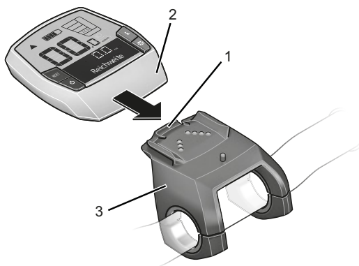
Rysunek 82: Wsunąć ekran (2) przez blokadę ekranu (1) do oporu w uchwyt (3)
