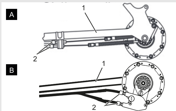
Rysunek 98: Nakrętki regulacyjne (2) w dwóch alternatywnych wersjach (A lub B) dwuczęściowego mechanizmu zmiany przerzutek na rurze dolnej tylnego trójkąta (1)
