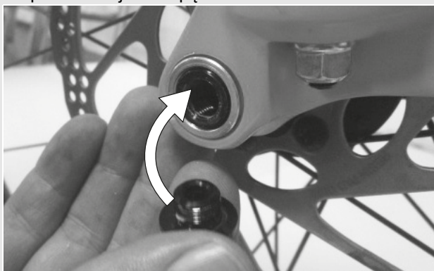
Rysunek 30: Sposób wsuwania dźwigni zacisku szybkoocucjącego w oś
