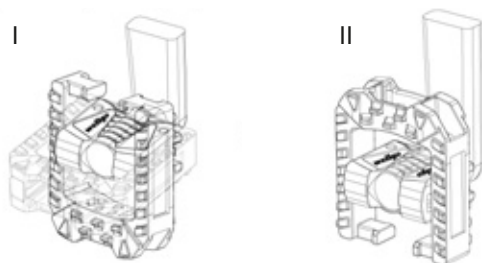
Rysunek 70: Ustawić pedał w pozycji dolnej (I) lub górnej (II)
