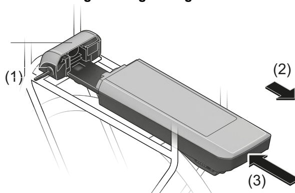
Rysunek 78: Wymywanie (2) i wkładanie (3) akumulatora zintegrowanego z bagażnikiem
