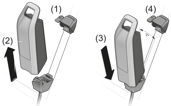
Obr. 29: Vyjmutí a vložení akumulátoru do rámu
