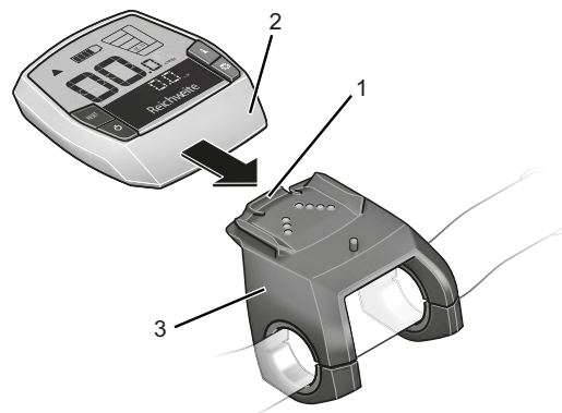
Obr. 34: Displej (2) přes aretaci displeje (1) posuňte až k dorazu držáku (3)
