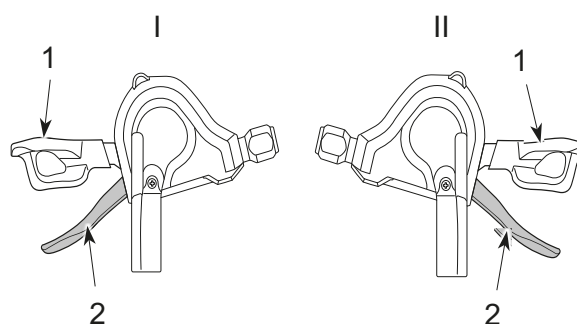
Obr. 36: Řadící páčka dolů (1) a řadící páčka nahoru (2) levého (I) a pravého (II) řazení
