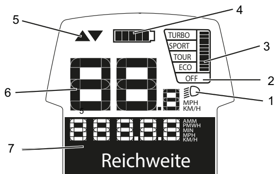
Obr. 18: Přehled ukazatelů na displeji
