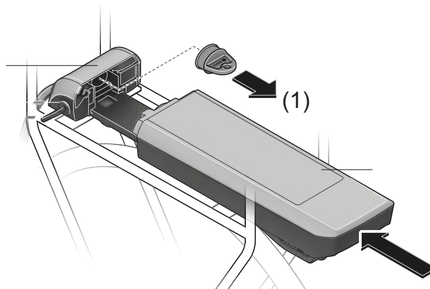
Obr. 33: Otevřené kontakty uzavřete krytkou, příklad nosiče zavazadel
