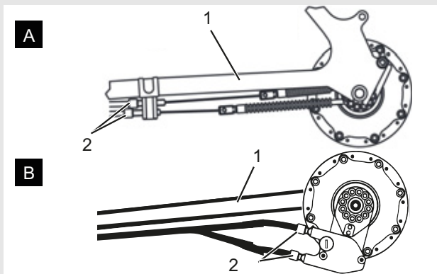
Obr. 41: Nastavovací pouzdra (2) řazení převodů ve dvou alternativních provedeních (A, resp. B) s ovládním dvěma lanky na zadní rámové stavbě (1)
