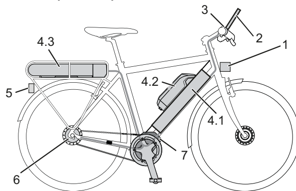
Obr. 6: Schéma elektrického hnacího systému
