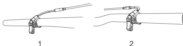
Obr. 24: Páka sedlovky namontovaná buď vlevo (1), nebo vpravo (2) na řídkách
