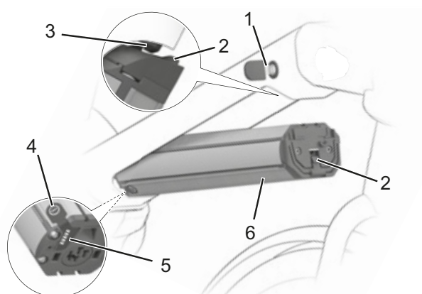
Obr. 11: Podrobnosti k integrovanému akumulátoru
