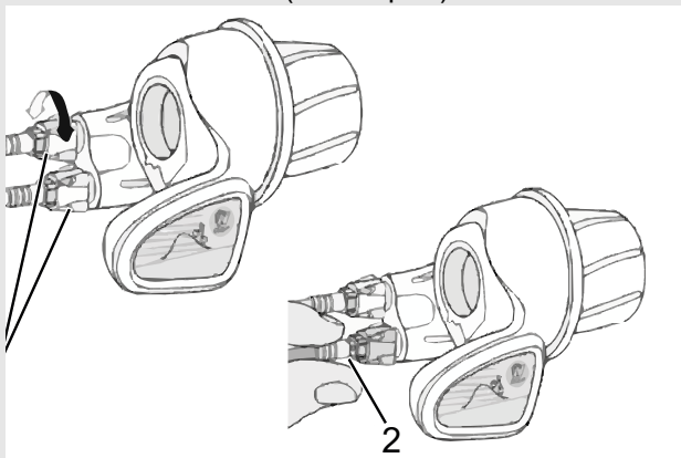
Obr. 42: Otočné řazení s nastavovacími pouzdry (1) a vůle řazení převodů (2)
