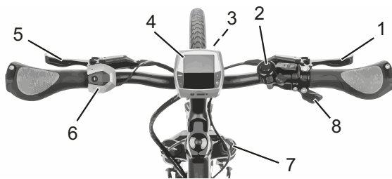
Obr. 14: Detail řídítek z pohledu jezdce, příklad
