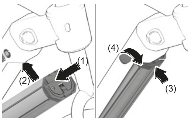
Obr. 32: Vložení integrovaného akumulátoru
