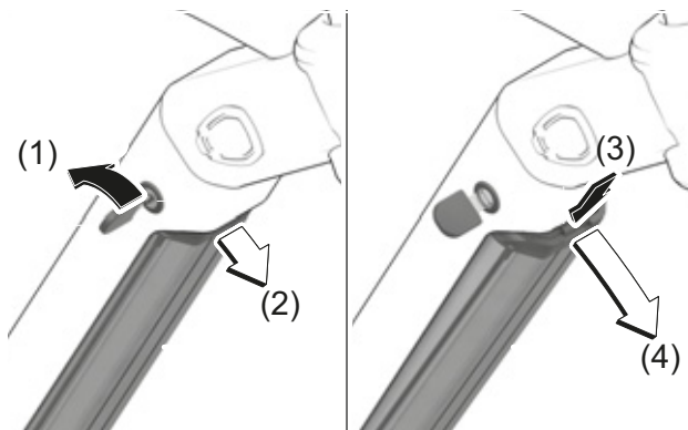
Obr. 31: Vyjmutí integrovaného akumulátoru
