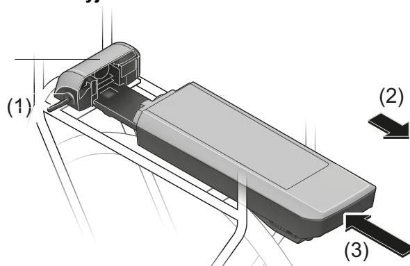
Obr. 30: Sejmutí (2) a vložení (3) akumulátoru na nosiči zavazadel
