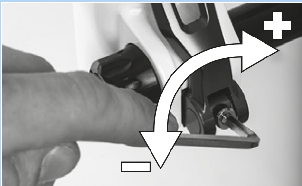
Obr. 153: Nastavení upínací síly rychloupínáku
