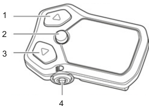
Obr. 38: Palubní počítač SHIMANO SC-E5003
