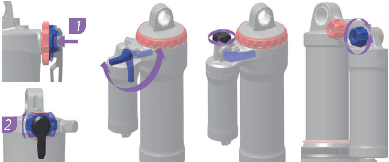
Obr. 230: Poloha a tvar nastavovacího šroubu komprese (modrý) jsou závislé na modelu
