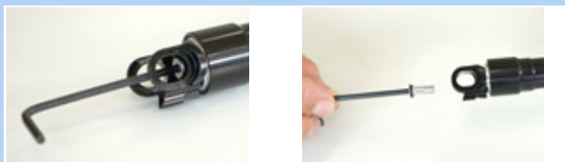
Obr. 175: Vyšroubování čepičky ventilku
