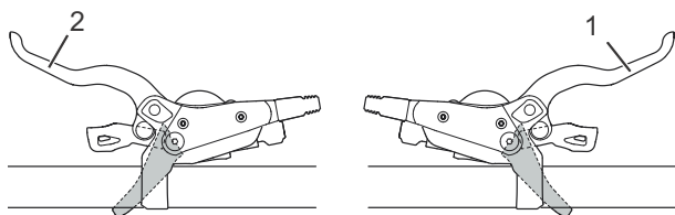
Obr. 129: Páka zadní (1) a přední brzdy (2), např. brzdy SHIMANO
