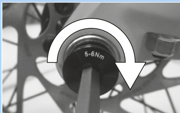
Obr. 53: Utažení pojistného šroubu
