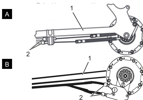
Obr. 150: Nastavovací pouzdra (2) řazení převodů ve dvou alternativních provedeních (A a B) s ovládním dvěma lanky na zadní rámové stavbě (1)
