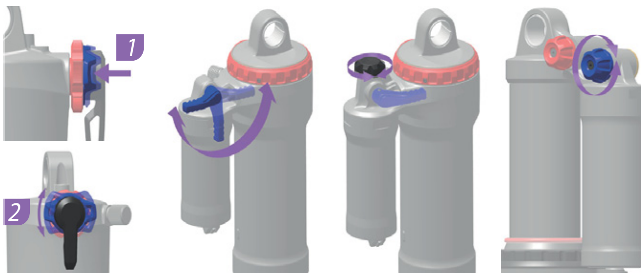
Obr. 106: Poloha a tvar nastavovacího šroubu komprese (modrý) jsou závislé na modelu
