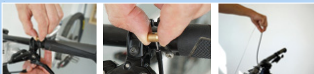
Obr. 194: Uvolnění dálkového ovládání
