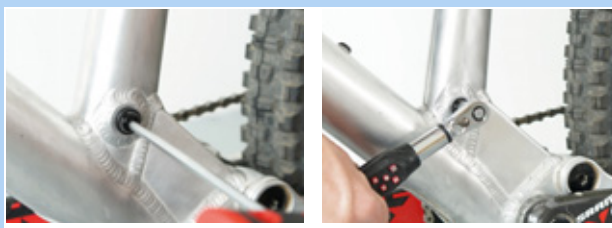
Obr. 216: Upevnění sedlovky
