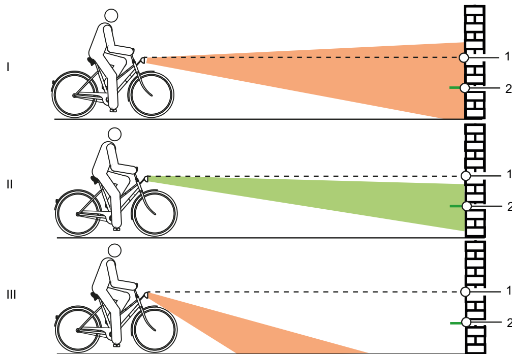
Obr. 145: Světlo nastavené příliš vysoko (1), správně (2) a příliš nízko (3)
