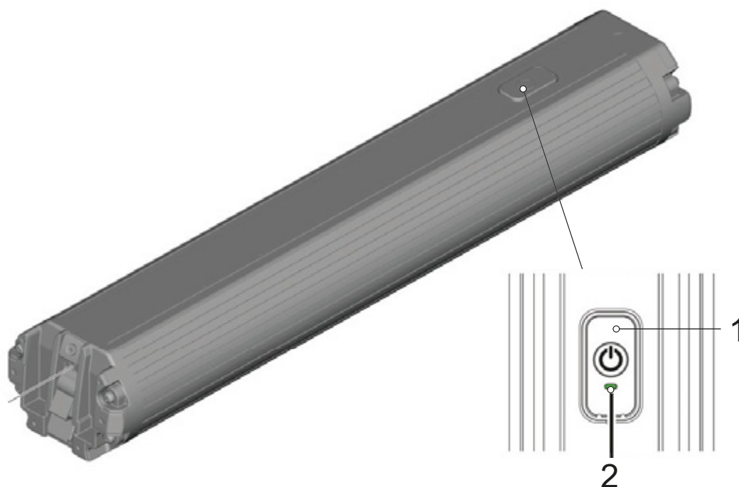
Obr. 46: Přehled akumulátorů SHIMANO BT-E8036
