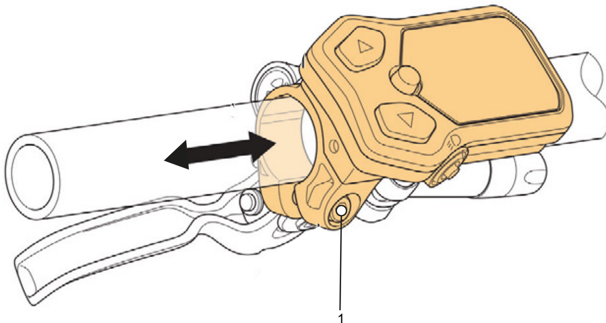
Obr. 96: Poloha upevňovacího šroubu palubního počítače SC-E5003
