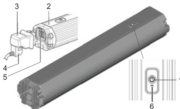
Obr. 35: Přehled akumulátorů SHIMANO BT-E8036
