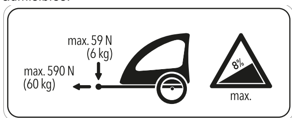
Figura 112: Placa indicadora de remolque
