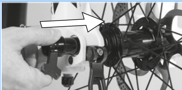
Figura 54: Inserción del eje transversal en la dirección de la flecha
