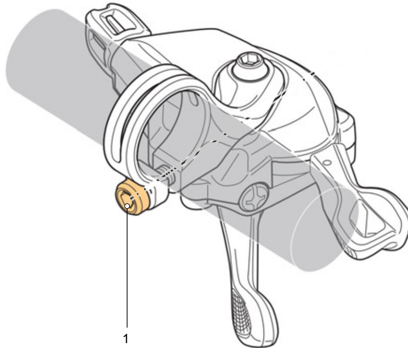
Figura 95: Posición del tornillo de fijación de la palanca de cambio SHIMANO
