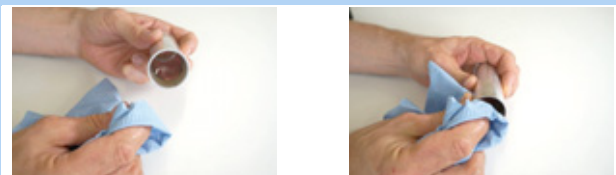
Figura 170: Limpieza del tubo del casquillo deslizante
