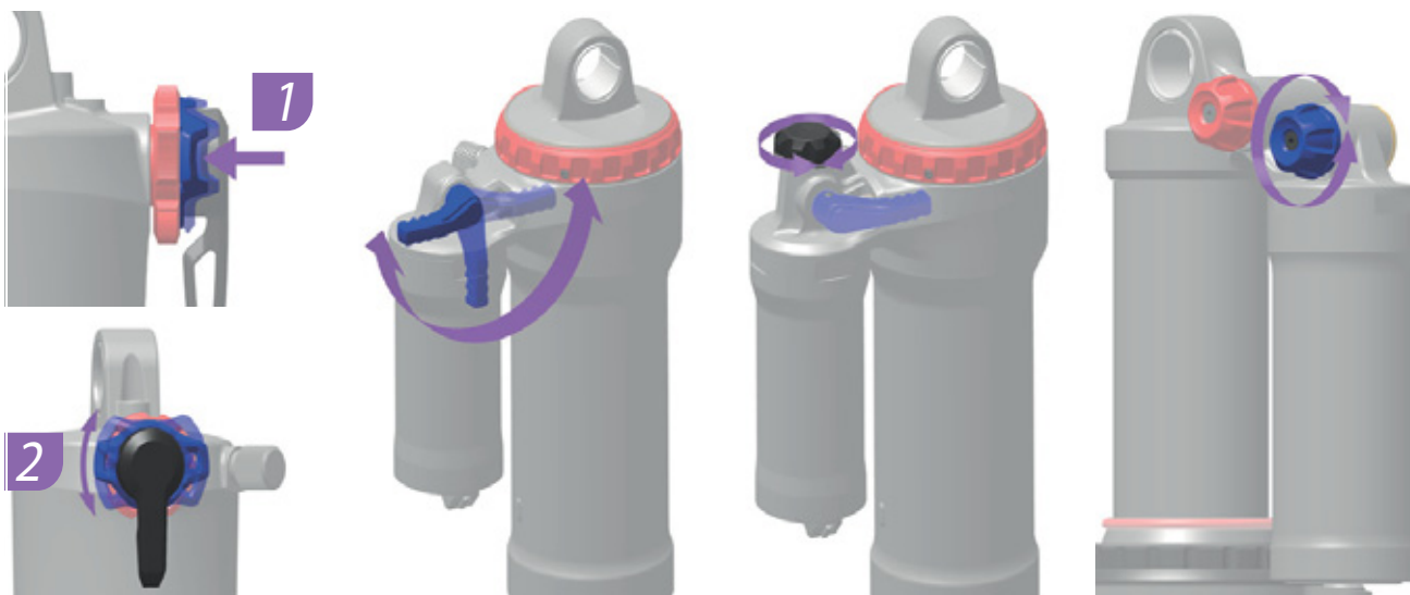
Figura 106: La posición y la forma del regulador de niveles de presión (azul) dependen del modelo
