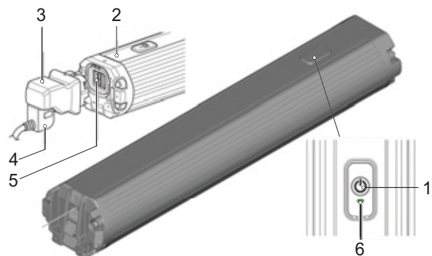
Figura 35: Vista general de la batería SHIMANO BT-E8036
