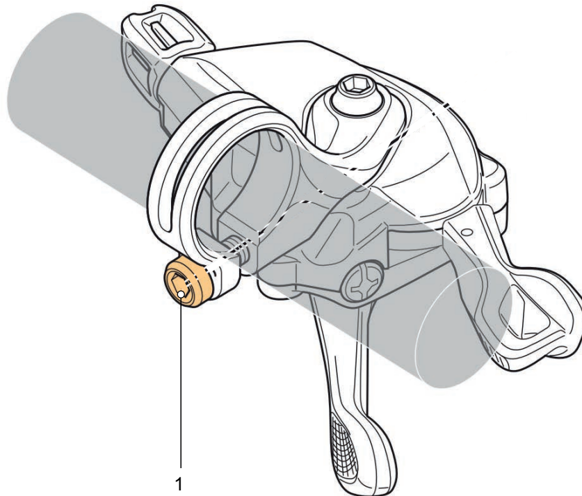
Abbildung 101: Lage Befestigungsschraube Schalthebel SHIMANO
