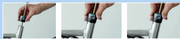
Abbildung 183: Außenhülse aufstecken
