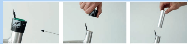
Abbildung 193: Außenhülse und Gleitbuchse ausbauen
