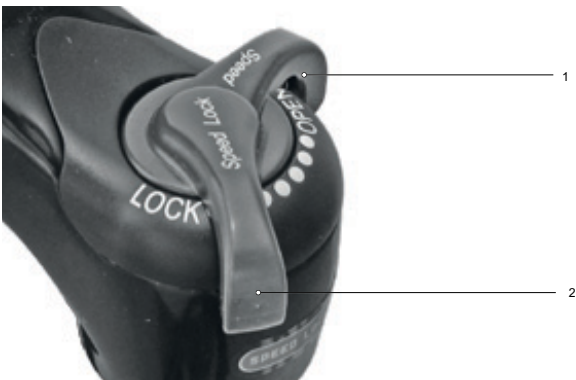
Abbildung 218: Druckstufeneinsteller härter einstellen
