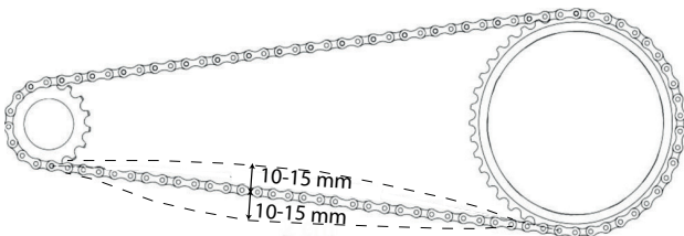
Abbildung 143: Kettenspannung prüfen
