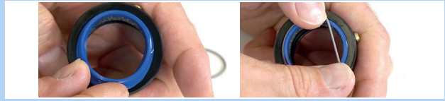
Abbildung 200: Abstreifer einlegen und befestigen
