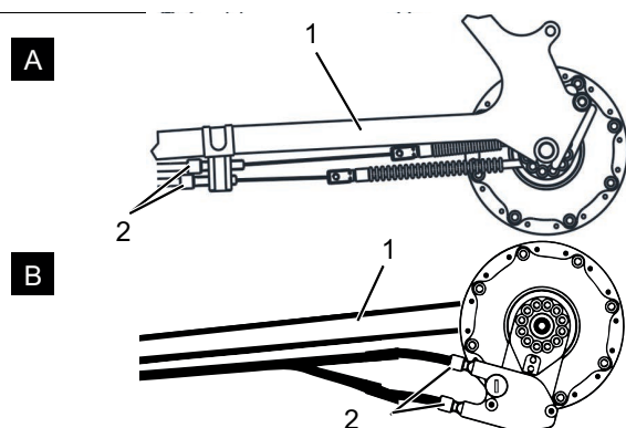
Abbildung 146: Einstellhülsen (2) an zwei alternativen Ausführungen (A und B) einer zweizügigen, seilzugbetätigten Gangschaltung an der Kettenstrebe (1)
