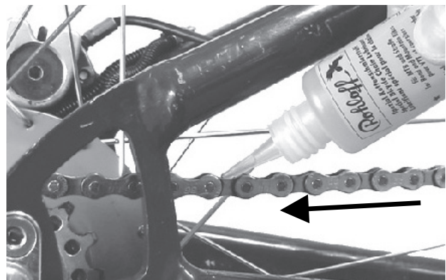
Abbildung 136: Kette schmieren
