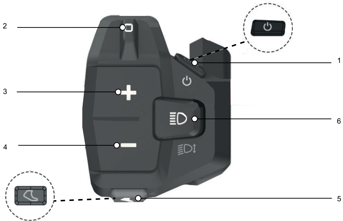
Abbildung 46: Übersicht Bedieneinheit BOSCH
