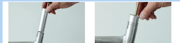
Abbildung 182: Gleitbuchsenrohr ins Sattelrohr stecken
