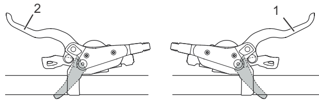
Figura 127: Palanca de freno trasero (1) y delantero (2), ejemplo freno SHIMANO
