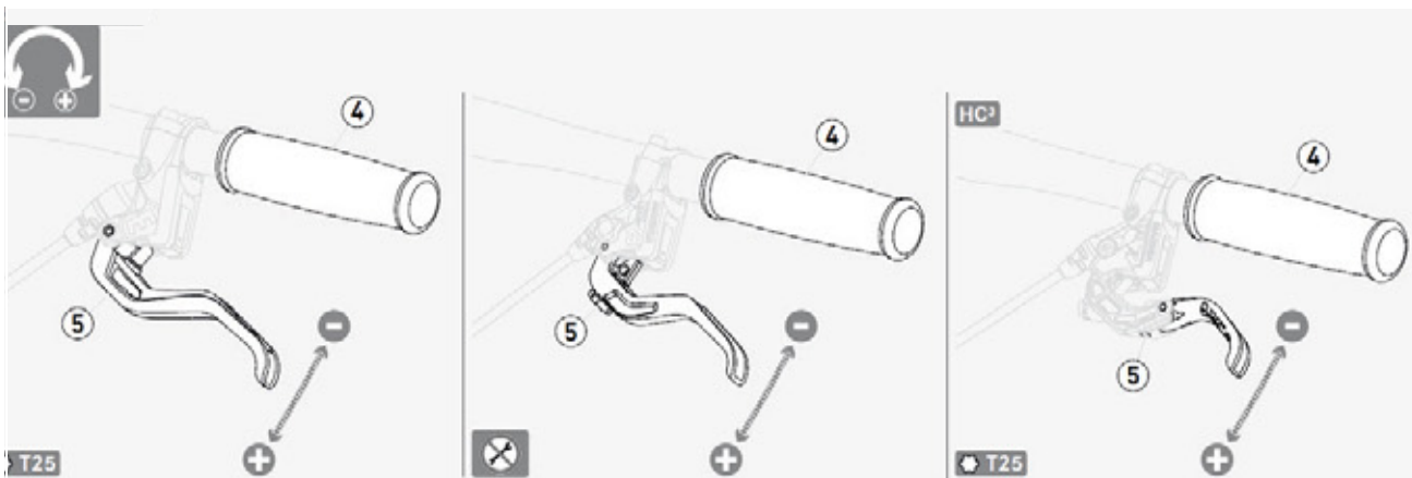
Figura 103: Ajuste del ancho de agarre de la palanca de freno con freno de disco MAGURA
