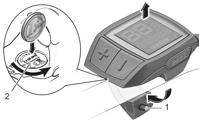
Figura 126: Ordenador de a bordo con tornillo de fijación (1) y tapa del compartimento de la batería (2)
