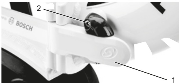
Figura 136: Palanca tensora del cuadro cerrada (1) y palanca de seguridad del cuadro cerrada (2)
