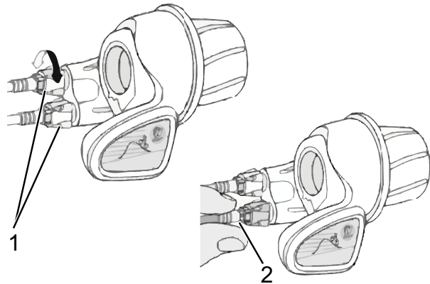
Figura 155: Puño giratorio con casquillos de ajuste (1) y holgura del cambio de marchas (2)
