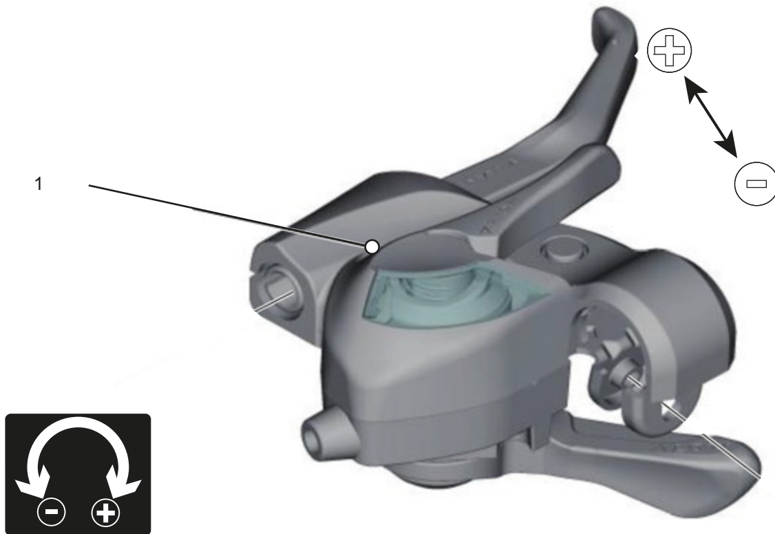
Figura 104: Posición del tornillo de ajuste (1)
