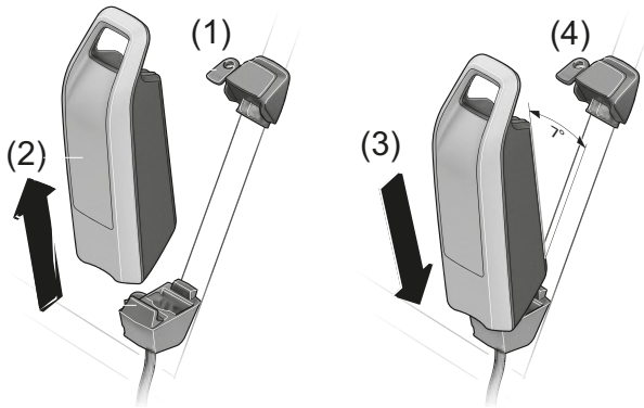
Figura 120: Extracción e inserción de la batería en el cuadro
