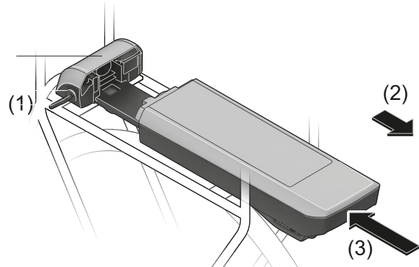
Figura 121: Extracción (2) e inserción (3) de la batería del portaequipajes
