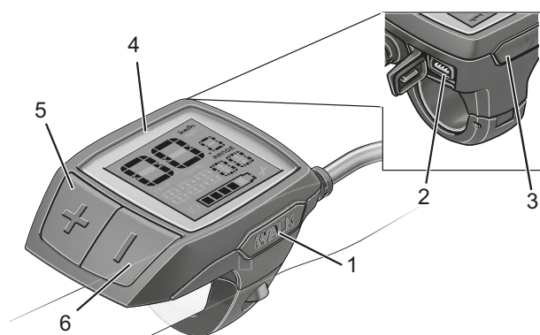
Figura 112: Estructura del ordenador de a bordo BOSCH Purion
