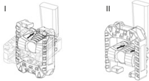
Figura 132: Plegado del pedal hacia abajo (I) o hacia arriba (II)
