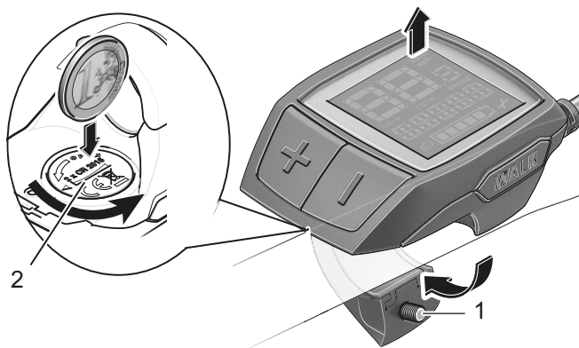
Illustration 126 : Ordinateur de bord avec vis de fixation (1) et couvercle du logement des piles (2)
