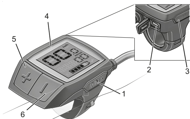
Illustration 125 : Structure de l'ordinateur de bord BOSCH Purion
