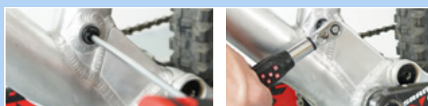
Illustration 191 : Fixer l'axe Postpin
