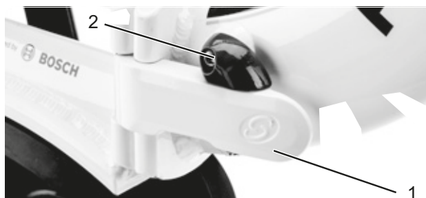
Illustration 138 : Levier de serrage du cadre fermé (1) et levier de blocage du cadre fermé (2)
