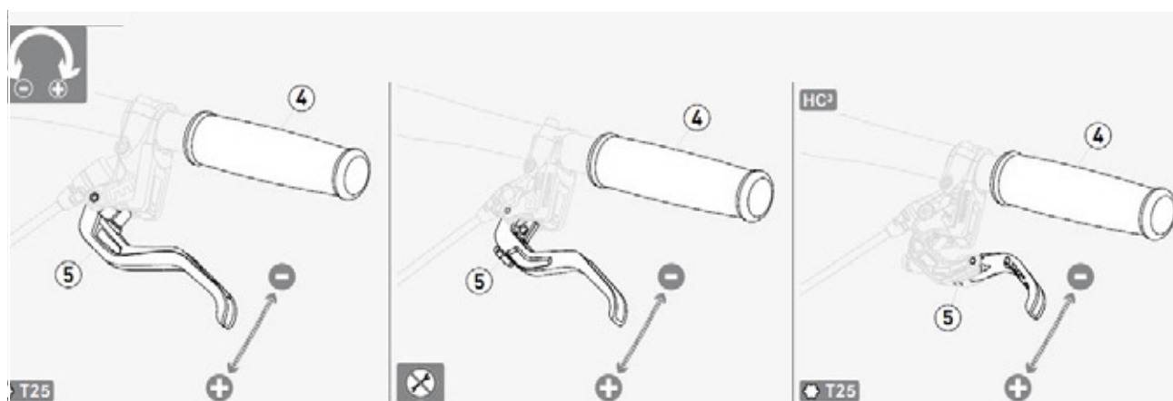
Illustration 103 : Régler la garde d'un levier de frein à disque MAGURA
