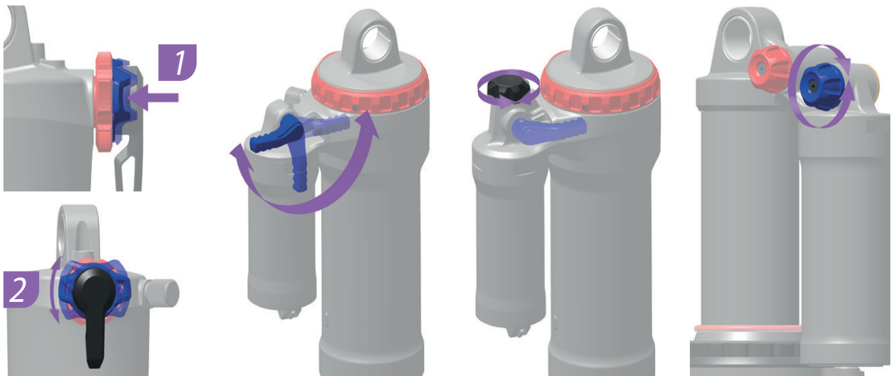
Abbildung 111: Lage und Form des Druckstufeneinstellers (blau) ist Modellabhängig
