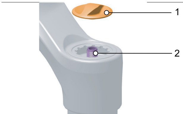
Abbildung 101: Abdeckung (1) von Luftventil (2) entfernen
