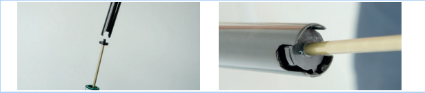
Abbildung 201: Höhenverstellungsklemme einfädeln
