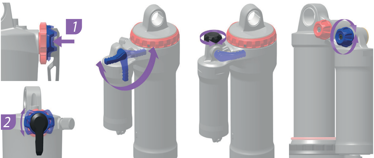
Abbildung 244: Lage und Form des Druckstufeneinstellers (blau) ist Modellabhängig
