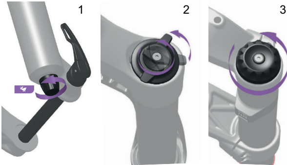
Abbildung 100: Zugstufe (1) und Druckstufendämpfer (2 und 3) öffnen
