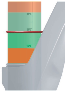
Abbildung 103: Vorgeschriebener SAG Bereich (grün) und verbotener AG Bereich (rot)
