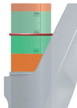
Abbildung 88: Vorgeschriebener SAG Bereich (grün) und verbotener SAG Bereich (rot)
