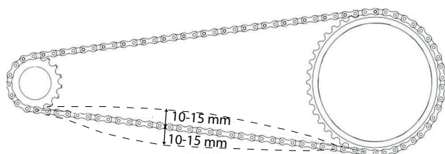
Abbildung 159: Kettenspannung prüfen
