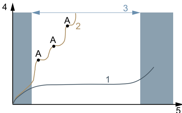
Abbildung 151: Diagramm Verschleiß, Betriebsdauer (x) zu Werstoffabtrag (y)
