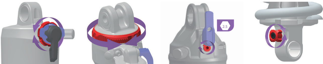
Abbildung 109: Lage und Form des Zugstufeneinstellers (rot) ist abhängig vom Modell
