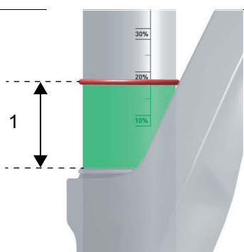
Abbildung 87: SAG (1)
