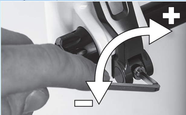
Abbildung 165: Spannkraft des Schnellspanners einstellen
