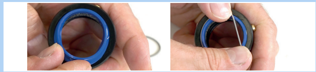
Abbildung 216: Abstreifer einlegen und befestigen
