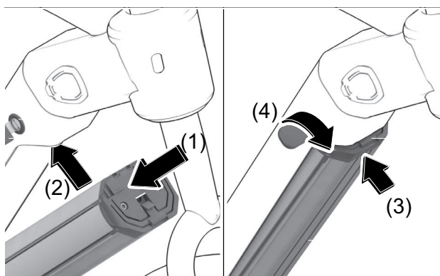
Abbildung 135: Akku einsetzen
