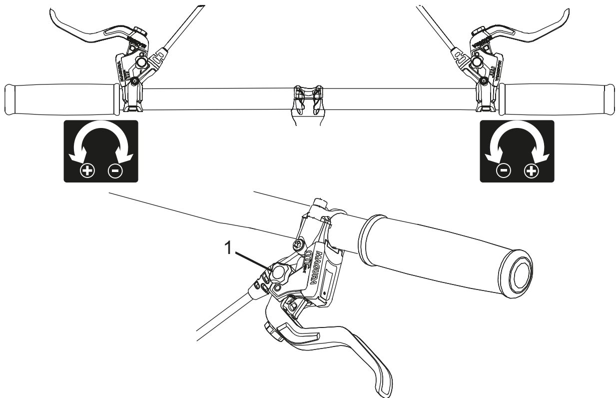
Rysunek 106: Ustawianie siły nacisku za pomocą gałki obrotowej (1)
