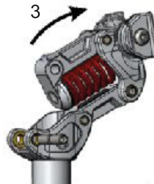
Rysunek 81: Pociągnąć górną część do przodu
