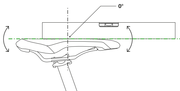
Rysunek 79: Poziome ustawienie siodełka z nachyleniem 0° jego środkowej części
