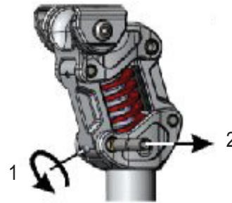
Rysunek 80: Wykręcić wkręt bez łba (1), po czym wyjąć oś ze stali nierdzewnej (2)
