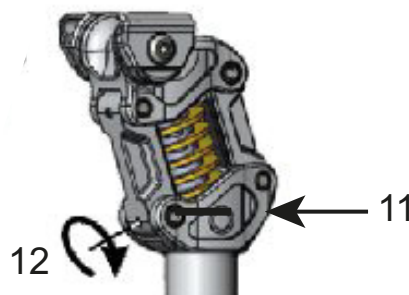
Rysunek 85: Nasmarować oś ze stali nierdzewnej (11) i dokręcić wkręt bez łba mocujący
