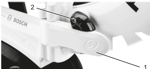
Rysunek 142: Zamknięta dźwignia mocująca (1) ramy i zamknięta dźwignia zabezpieczająca (2) ramy
