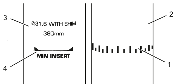
Rysunek 76: Widok szczegółowy sztycy podsiodłowych, przykłady oznaczenia minimalnej głębokości osadzenia
