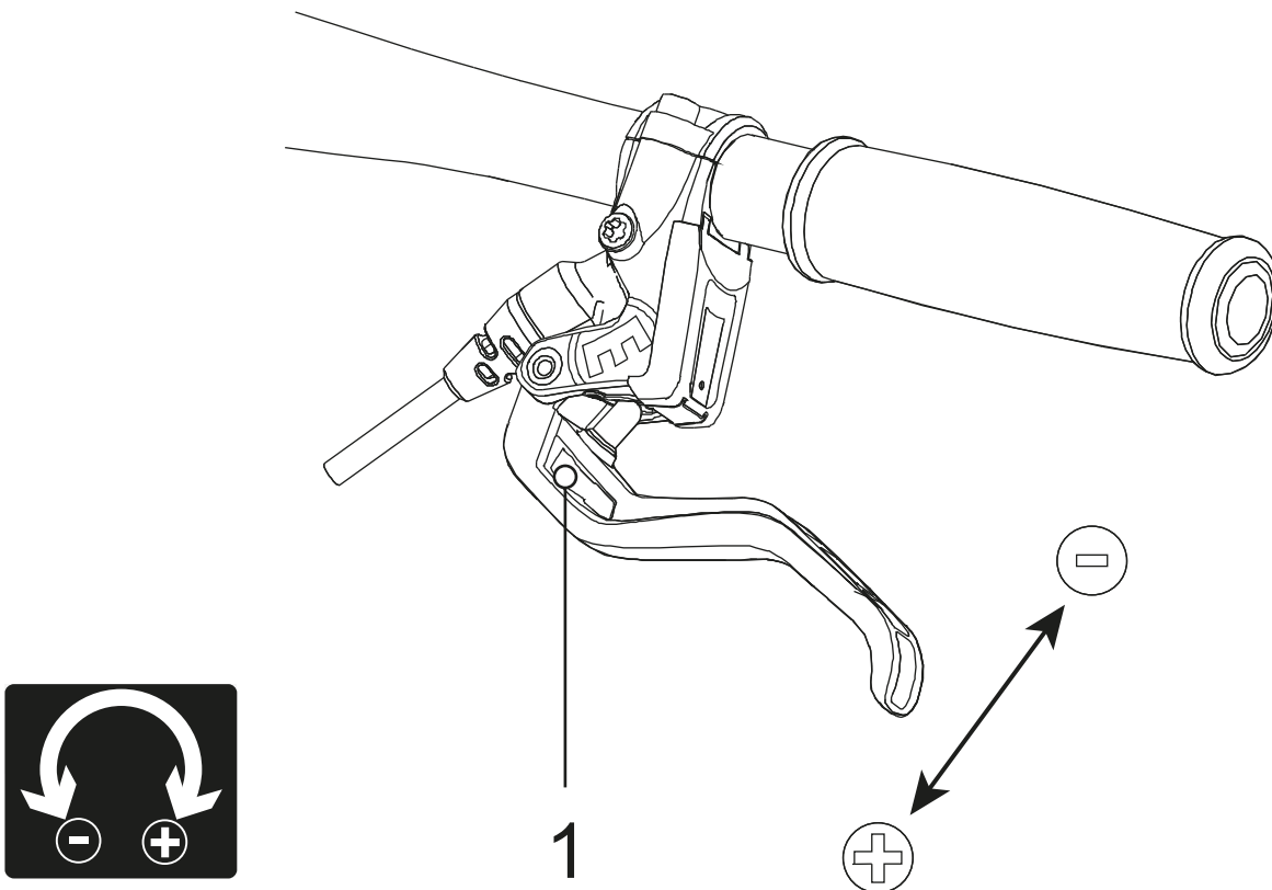
Rysunek 104: Ustawianie odchylenia manetki dźwigni hamulca MAGURA HS 33
