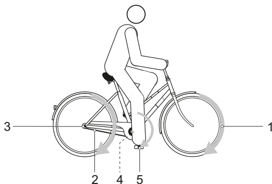
Rysunek 28: Schemat mechanicznego układu napędowego
