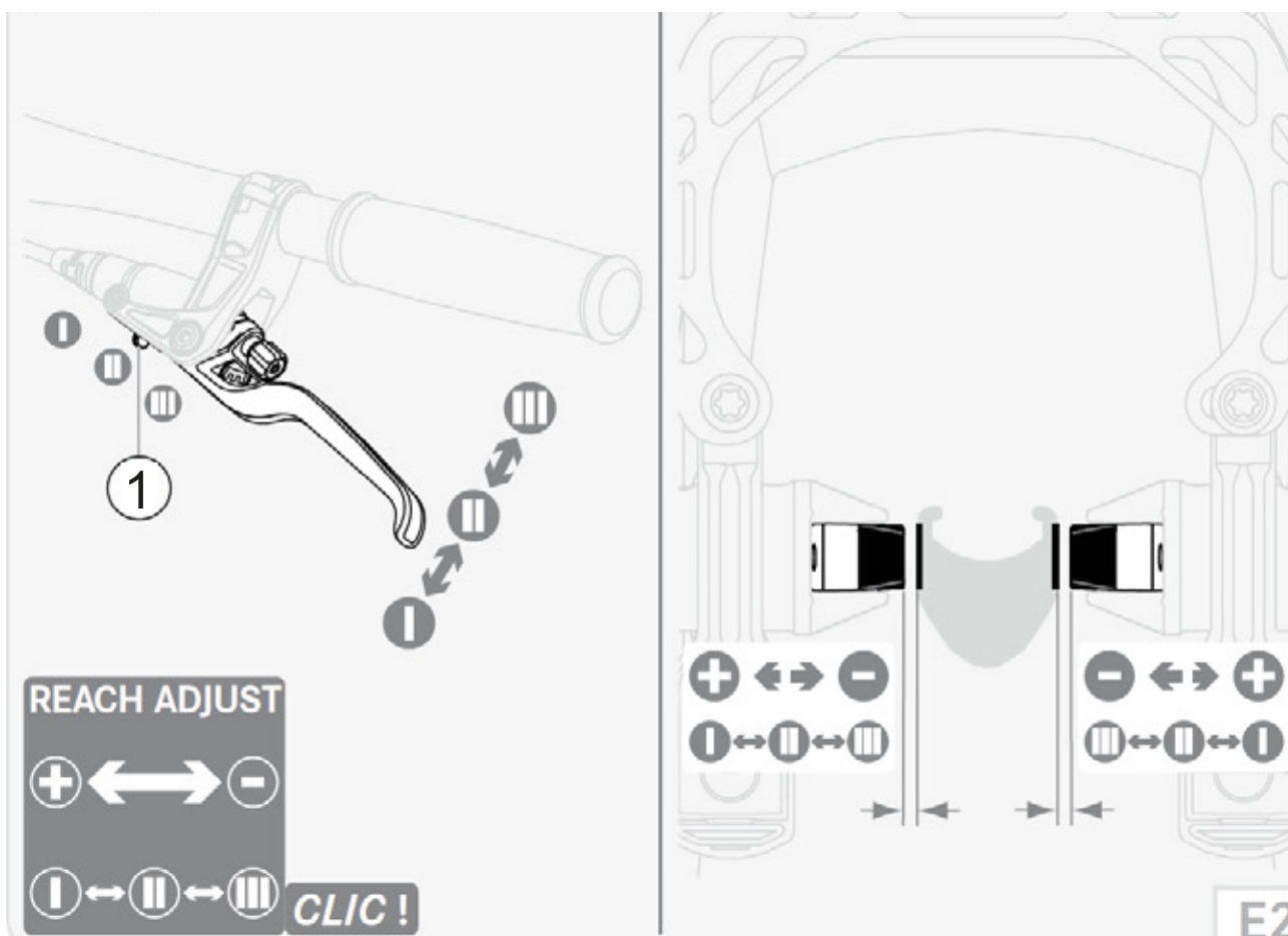
Rysunek 103: Ustawianie odchylenia manetki dźwigni hamulca MAGURA HS 22
