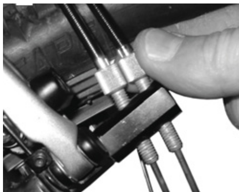
Rysunek 154: Wersje piast Rohloff z wewnętrznym sterowaniem zmiany biegów posiadają regulator naprężenia na wsporniku linek
