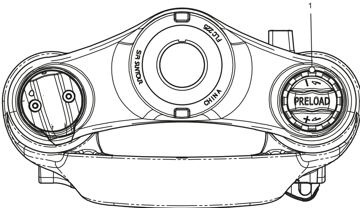
Rysunek 107: Pokrętko regulacyjne parametru SAG (1) usytuowane na koronie widelca amortyzowanego
