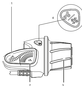
Rysunek 133: Manetka obrotowa ENVIOLo ze wskaźnikiem
