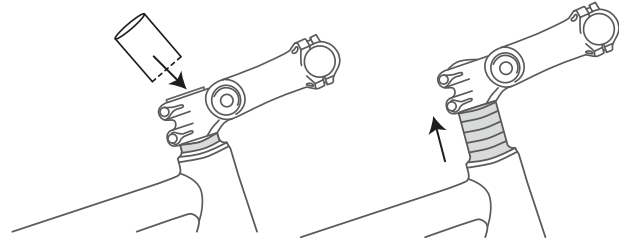
Rysunek 91: Podwyższanie mostka typu A-head przez montaż pierścieni dystansowych
