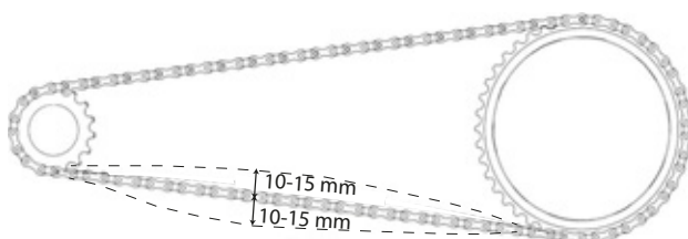
Rysunek 153: Kontrola naprężenia łańcucha
