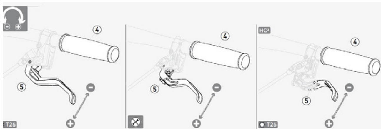
Rysunek 102: Ustawianie odchylenia manetki dźwigni hamulca tarczowego MAGURA
