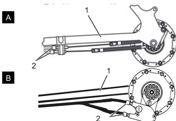
Rysunek 157: Nakrętki regulacyjne (2) w dwóch alternatywnych wersjach (A i B) dwuczętnowego mechanizmu zmiany przerzutek na rurze dolnej tylnego trójkąta (1)
