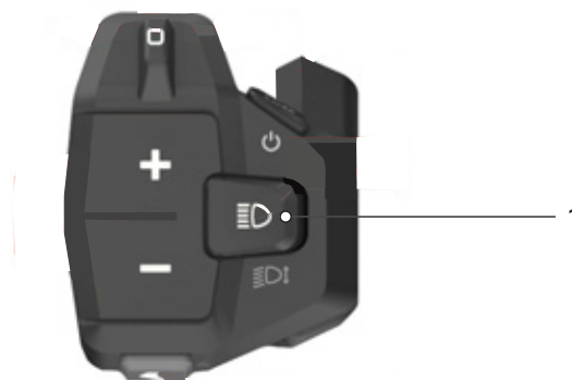
Rysunek 121: Położenie przycisku świateł do jazdy
