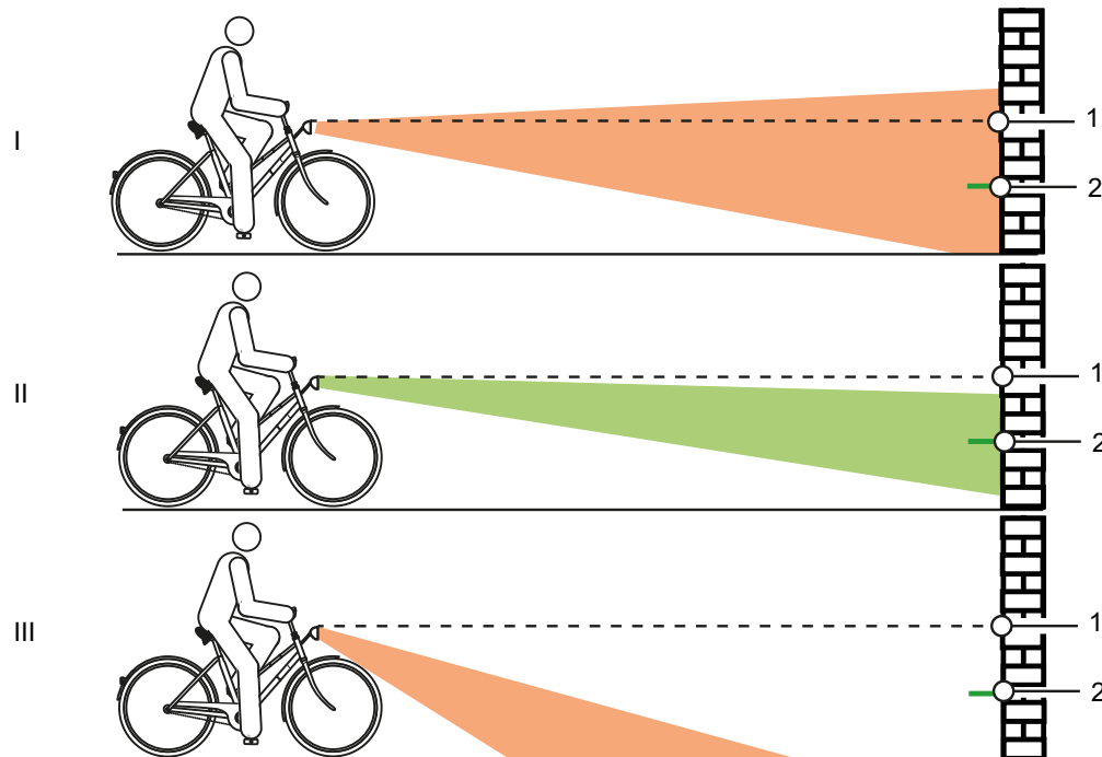
Rysunek 113: Światło ustawione za wysoko (1), prawidłowo (2) i za nisko (3)
