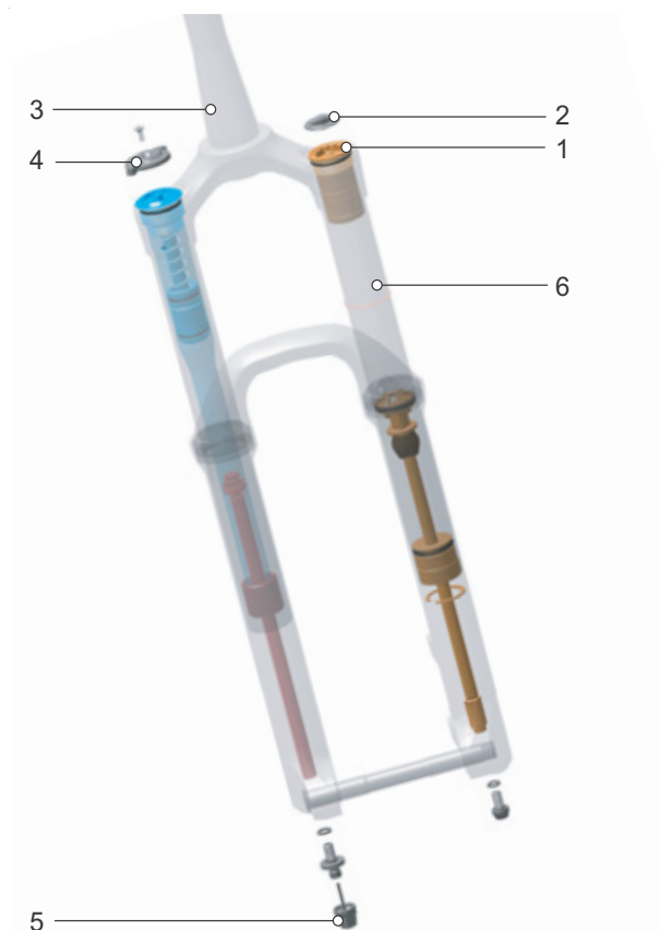
Rysunek 11: Budowa wewnętrzna widełca amortyzatora pneumatycznego
