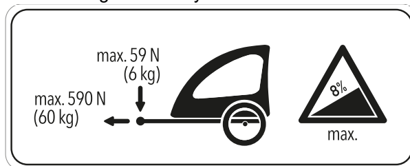
Rysunek 114: Tabliczka informacyjna przyczepki
