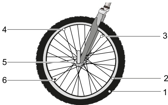
Afbeelding 22: Zichtbare componenten van het wiel
