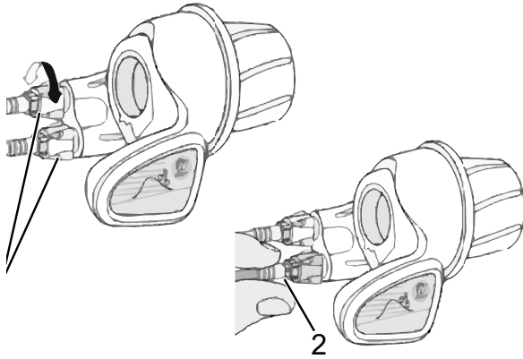
Afbeelding 198: Draaibare handvatschakelaar met afstelwartels (1) en speling van de versnelling (2)
