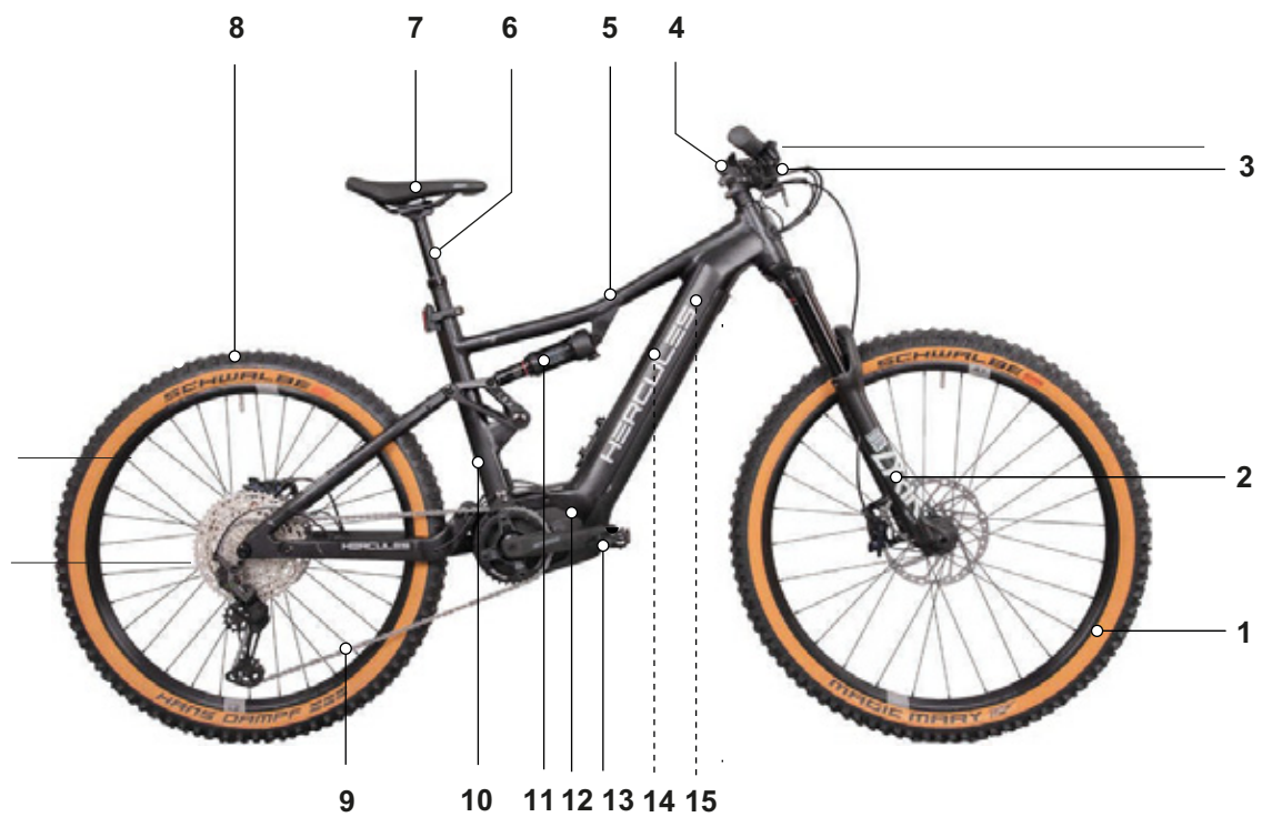
Afbeelding 3: Pedelec van rechts gezien, voorbeeld HERCULES NOS FS 1.1
