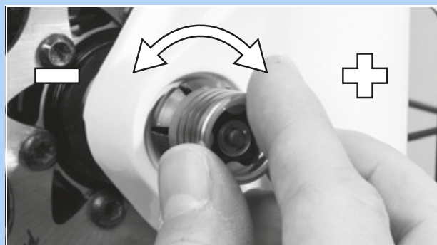
Afbeelding 83: Spanning afstellen
