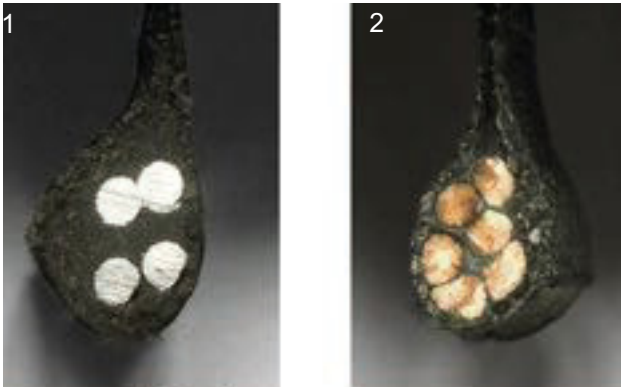
Afbeelding 25: draadkern (1) en Kevlarkern (2)
