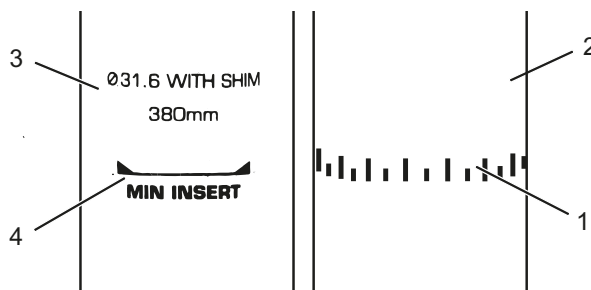
Afbeelding 109: Detailaanzicht zadelpen, voorbeelden van de markering van de minimale insteekdiepte
