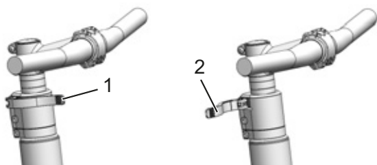
Afbeelding 115: Gesloten (1) en geopende (2) voorbouwspanhendel, voorbeeld All Up
