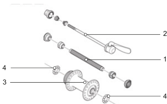
Afbeelding 30: Voorbeeld voorwielnaaf, SHIMANO
