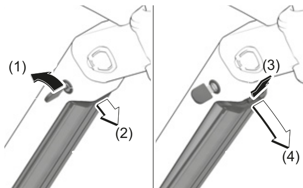
Afbeelding 149: Accu verwijderen
