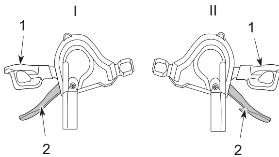
Figura 85: Palanca de cambio hacia abajo (1) y palanca de cambio hacia arriba (2) del cambio de marchas izquierdo (I) y derecho (II)
