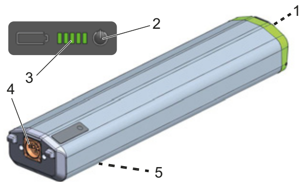
Figura 16: Detalle de la batería SuperCore
