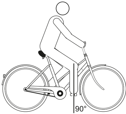
Figura 50: Plomada desde la rótula
