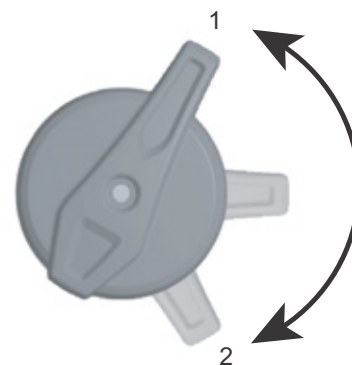
Figura 73: Regulador de niveles de presión FOX con las posiciones ABIERTO (1) y DURO (2)
