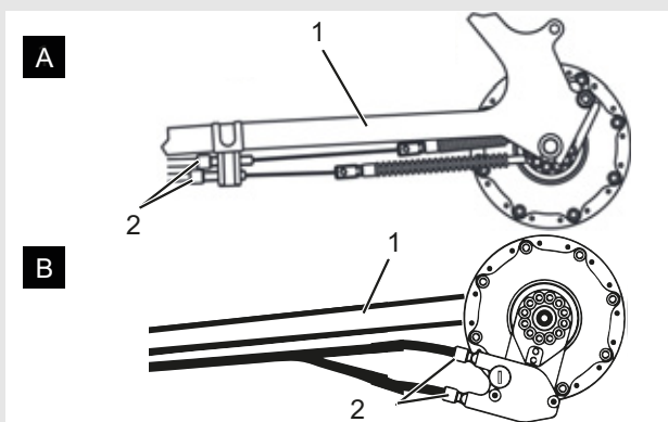
Figura 87: Casquillos de ajuste (2) en dos versiones alternativas (A o B) de un cambio de marchas accionado por cable de accionamiento, de dos cables en la vaina (1)
