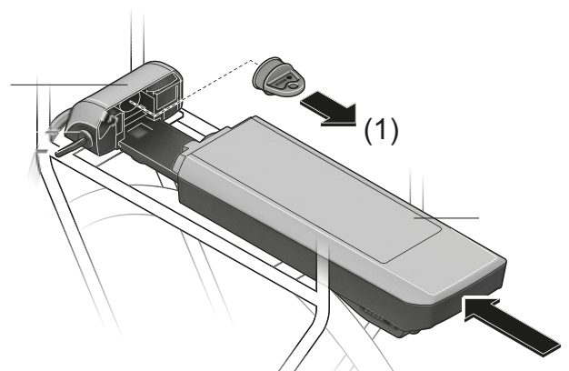
Figura 70: Cierre de los contactos abiertos con tapa de cierre, ejemplo batería del portaequipajes
