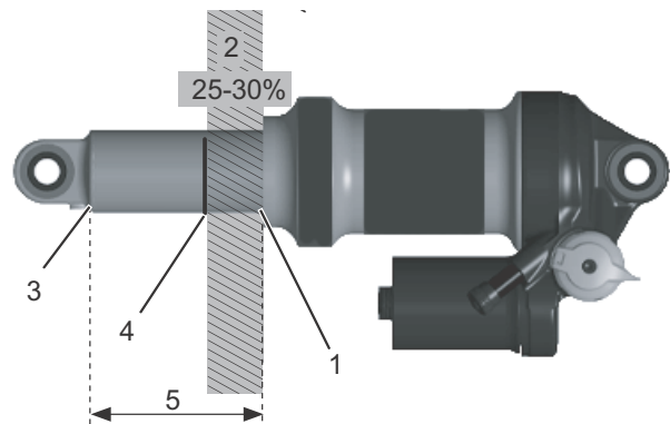
Figura 63: Amortiguador de la horquilla trasera FOX:
