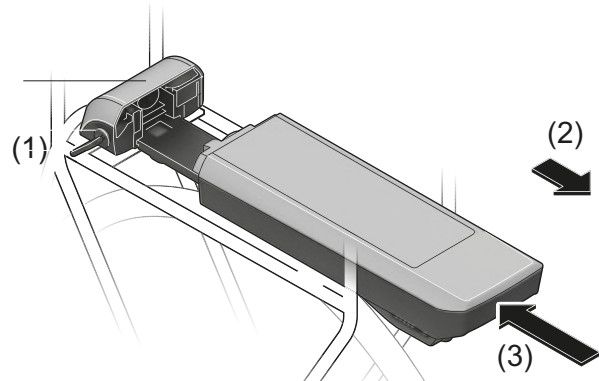
Figura 67: Extracción (2) e inserción (3) de la batería del portaequipajes
