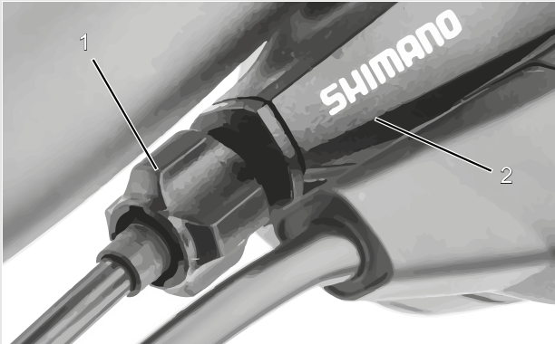
Figura 86: Casquillo de ajuste (1) del cambio de marchas accionado por cable de accionamiento con carcasa de la palanca de cambio (2), ejemplo
