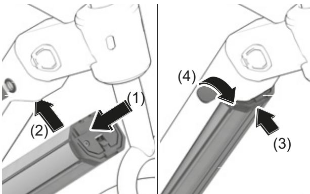
Figura 69: Inserción de la batería integrada
