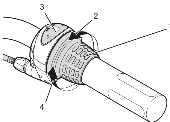
Figura 82: Ejemplo cambio de marchas Shimano Nexus: puño giratorio (1) del cambio de buje con su visualización (2), sentido de giro para aumentar la marcha (3) y el sentido de giro para reducir la marcha (4).
