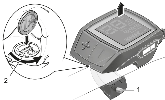
Figura 71: Pantalla con tornillo de fijación (1) y tapa del compartimento de la batería (2)
