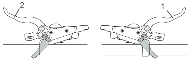
Figura 72: Palanca de freno detrás (1) y delante (2), ejemplo freno Shimano
