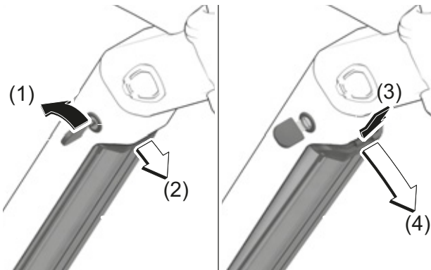
Figura 66: Extracción e inserción de la batería en el cuadro
