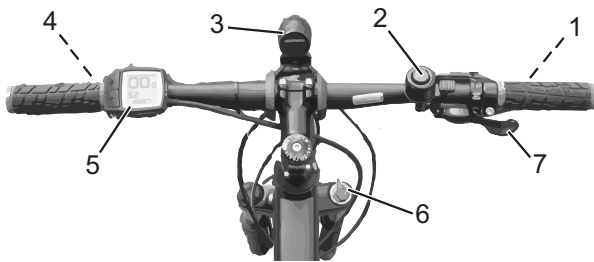
Figura 20: Vista detallada del Pedelec desde la posición del conductor, ejemplo
