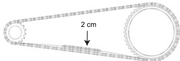
Illustration 71 : Contrôler la tension de la chaîne
