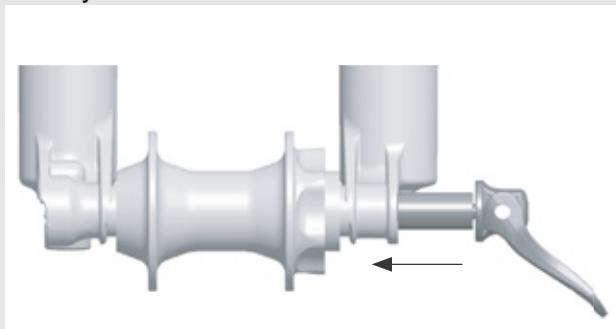
Illustration 36 : Enfoncez l'attache rapide
