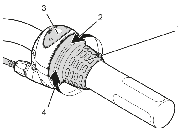
Illustration 70 : Exemple d'un changement de vitesse Shimano Nexus : Poignée de vitesse rotative (1) du moyeu à vitesses intégrées avec son affichage (3), le sens de rotation pour passer à une vitesse supérieure (2) et le sens de rotation pour une vitesse inférieure (4)
