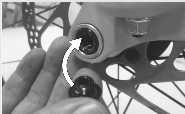
Illustration 22 : Enfoncer le levier d'attache rapide dans l'axe
