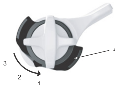
Illustration 63 : Le réglage fin de la position OUVERT se fait au moyen du dispositif de réglage (4)
