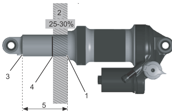
Illustration 57 : Structure d'un amortisseur arrière FOX
