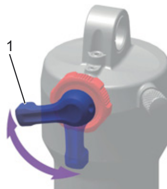
Illustration 68 : Régler la dureté de l'amortisseur de compression sur le levier (1) de l'amortisseur arrière
