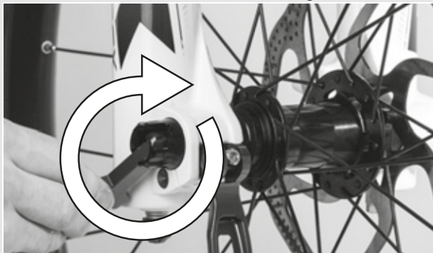
Illustration 27 : Serrer l'axe
