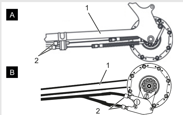
Illustration 75 : Douilles de réglage (2) sur deux modèles alternatifs (A et B) d'un changement de vitesse actionné par câble à deux câbles sur la base de cadre (1)
