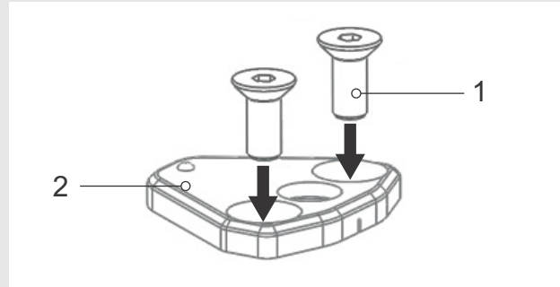
26. ábra: Süllyesztett fejű csavarok bedugása az alaplemezbe
