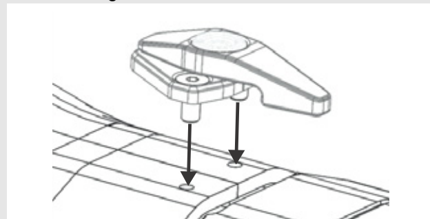
28. ábra: Kar csavarozása a vázra
