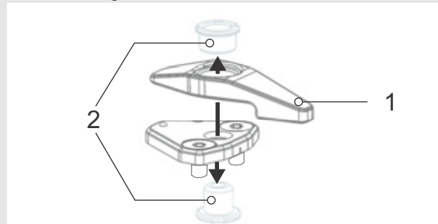
27. ábra: Rögzítőkar összekötése az alaplemezzel
