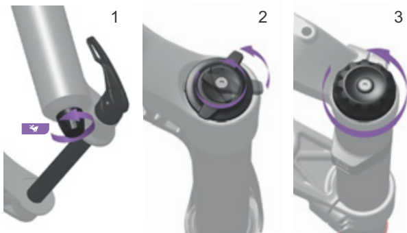
Afbeelding 99: Trekdemper (1) en drukdempers (2 en 3) openen
