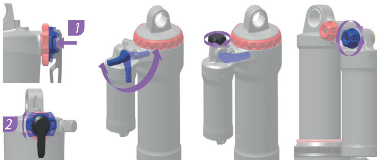
Afbeelding 110: Locatie en vorm van de drukdemperafsteller (blauw) is afhankelijk van het model
