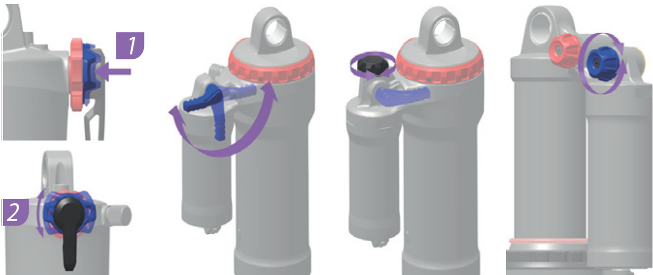
Afbeelding 243: Locatie en vorm van de drukdemperafsteller (blauw) is afhankelijk van het model
