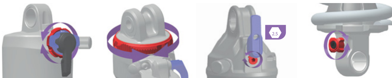
Afbeelding 239: Locatie en vorm van de trekdemperafsteller (rood) is afhankelijk van het model
