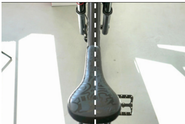
Afbeelding 62: Zadel in rijrichting uitlijnen
