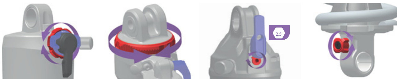
Afbeelding 237: Locatie en vorm van de trekdemperafsteller (rood) is afhankelijk van het model
