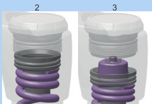
Afbeelding 98: Voorspanningsafstelring in- en uitdraaien
