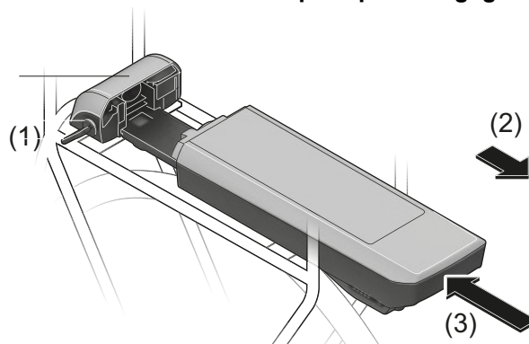
Illustration 78 : Retirer (2) et insérer (3) la batterie pour porte-bagages
