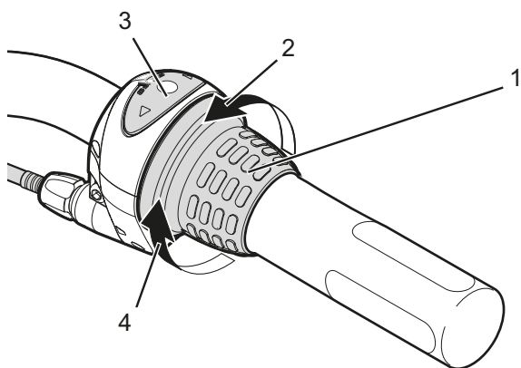
Illustration 93 : Exemple d'un changement de vitesse Shimano Nexus : Poignée de vitesse rotative (1) du moyeu à vitesses intégrées avec son affichage (3), le sens de rotation pour passer à une vitesse supérieure (2) et le sens de rotation pour une vitesse inférieure (4)
