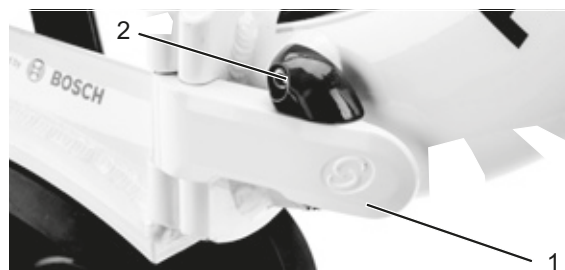
Illustration 74 : Cadre, avec levier de serrage du cadre fermé (1) et levier de blocage du cadre fermé (2) Déplier la pédale
