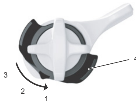
Illustration 86 : Le réglage fin de la position OUVERT se fait au moyen du dispositif de réglage (4)
