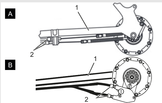
Illustration 98 : Douilles de réglage (2) sur deux modèles alternatifs (A et B) d'un changement de vitesse actionné par câble à deux câbles sur la base de cadre (1)
