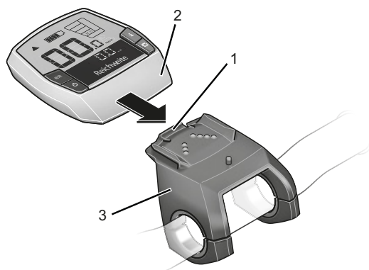
Illustration 82 : Enfoncer l'écran (2) via le dispositif de blocage de l'écran (1) jusqu'à la butée du support (3)
