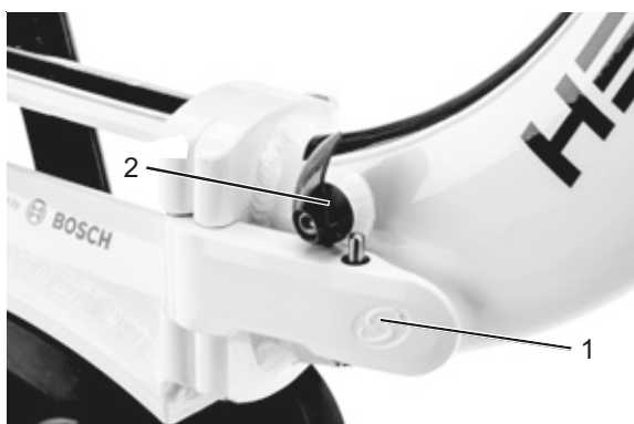
Illustration 73 : Cadre, avec levier de serrage du cadre fermé (1) et levier de blocage du cadre ouvert (2)
