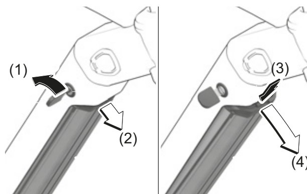
Illustration 79 : Retirer la batterie intégrée
