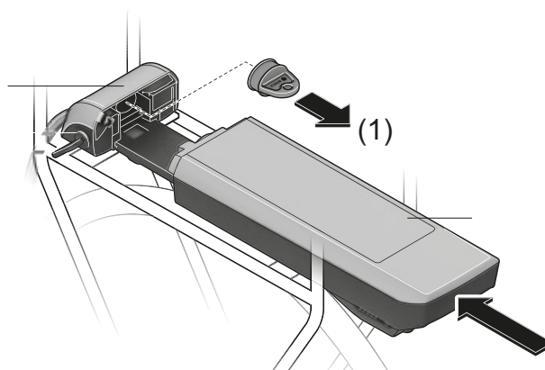
Illustration 81 : Couvrir les contacts ouverts avec un cache, exemple d'une batterie pour porte-bagages
