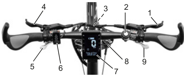
Figura 19: Particolare del pedelec visto dalla posizione del ciclista, esempio
