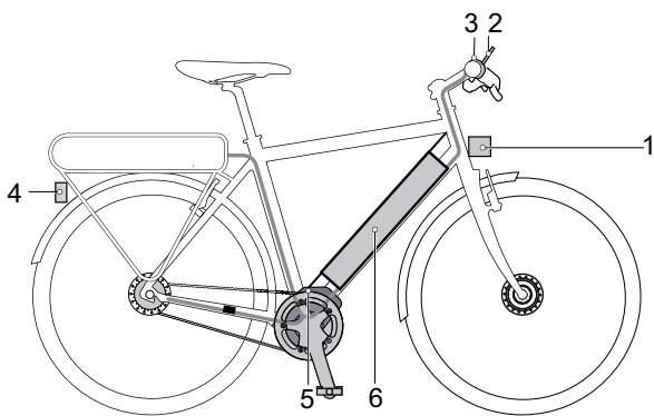
Abbildung 32: Schema Elektrisches Antriebssystem
