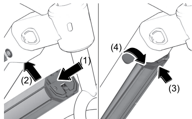
Abbildung 119: Akku einsetzen
