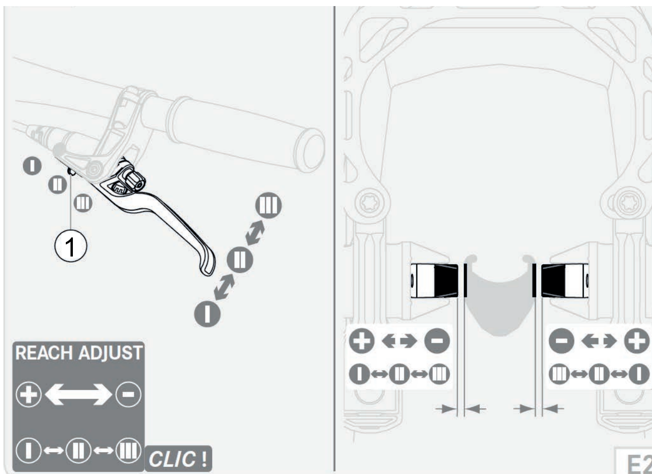
Abbildung 97: Griffweite Bremshebel MAGURA HS 22 einstellen
