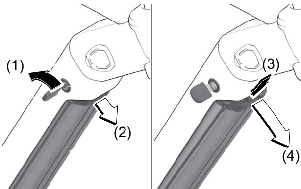
Abbildung 118: Akku herausnehmen
