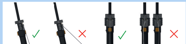
Abbildung 161: Korrekter und falscher Bowdenzug
