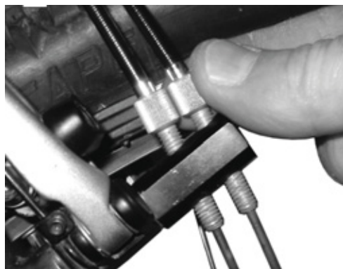
Obr. 150: Náboje Rohloff s vnitřním ovládním řazení mají nastavovače napnutí na držáku protitahu
