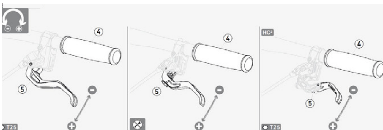
Obr. 103: Nastavení vzdálenosti brzdové páky kotoučové brzdy MAGURA
