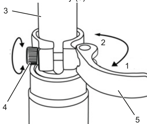
Obr. 83: Otevření rychloupínáku sedlovky
