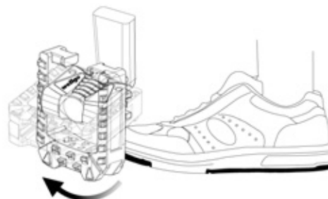
Obr. 138: Složení pedálu směrem nahoru
