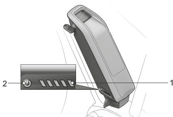
Obr. 43: Poloha indikátoru stavu nabití akumulátoru v rámu
