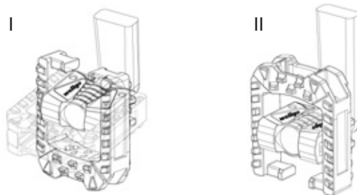
Obr. 132: Složení pedálu směrem dolů (I) nebo nahoru (II)
