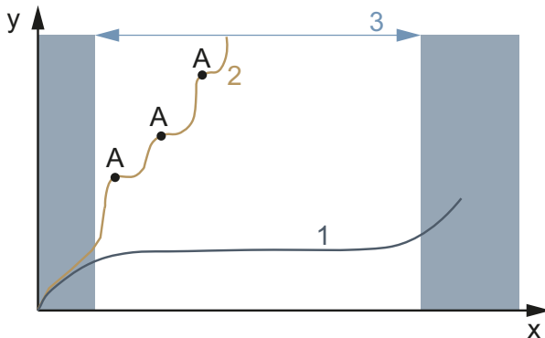
Obr. 142: Diagram opotřebení, provozní životnost (x) v závislosti na opotřebení materiálu (y)
