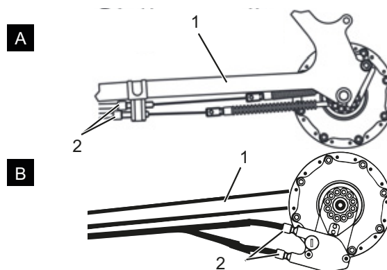
Obr. 153: Nastavovací pouzdra (2) řazení převodů ve dvou alternativních provedeních (A a B) s ovládním dvěma lanky na zadní rámové stavbě (1)
