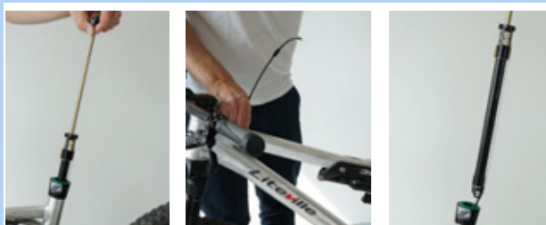
Obr. 162: Vytážení kazety
