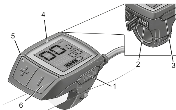
Obr. 125: Struktura palubního počítače BOSCH Purion
