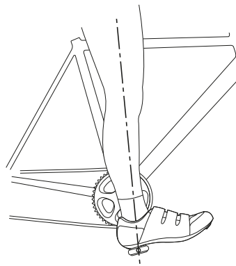
Obr. 82: Metoda podpatku
