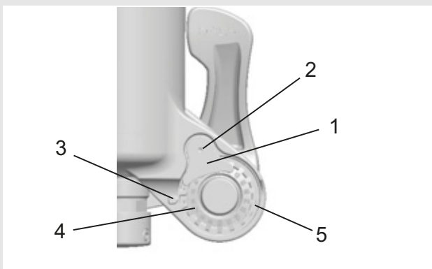
Figura 50: Vista posteriore della struttura del bloccaggio rapido con sicura del dado dell'asse (1) e dado dell'asse (5)
