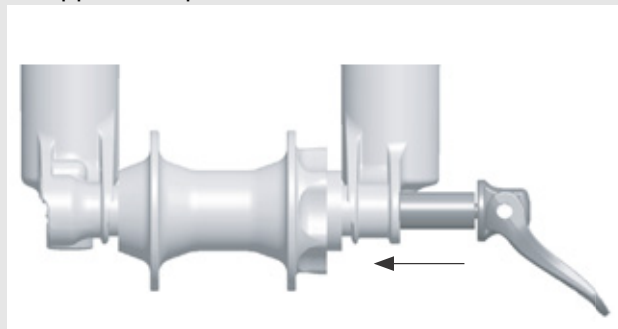
Figura 48: Inserimento del bloccaggio rapido
