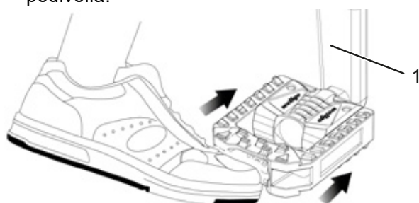
Figura 79: Spinta del pedale contro la pedivella (1)
