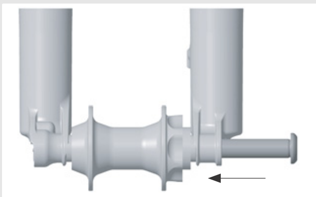
Figura 51: Inserimento dell'asse Kabolt
