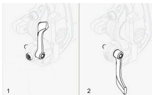
Figura 9: Leva di bloccaggio del freno a pattino, chiusa (1) e aperta (2)
