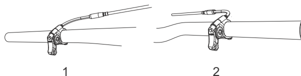
Figura 56: Leva del canotto reggisella montata a sinistra (1) o a destra (2) sul manubrio
