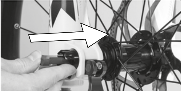
Figura 40: Applicazione della leva del bloccaggio rapido nel perno
