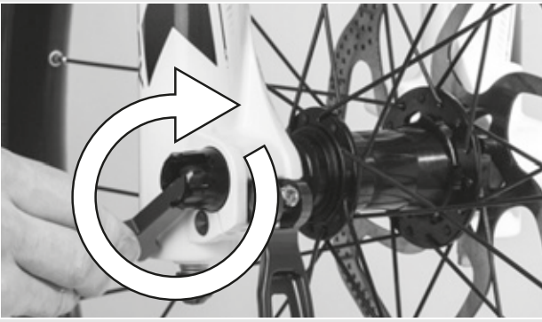
Figura 39: Serraggio del perno
