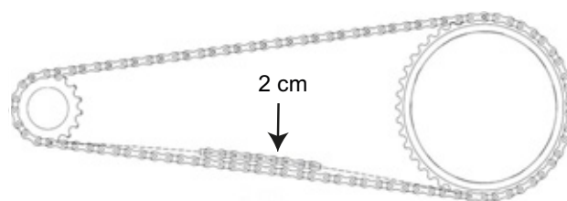
Figura 87: Controllo della tensione della catena
