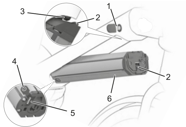
Figura 17: Dettaglio della batteria integrata
