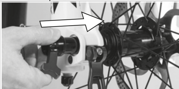
Figura 38: Applicazione del perno nel mozzo
