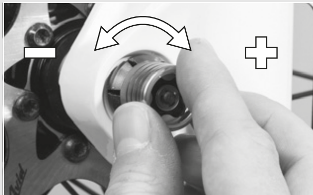
Figura 46: Regolazione del serraggio
