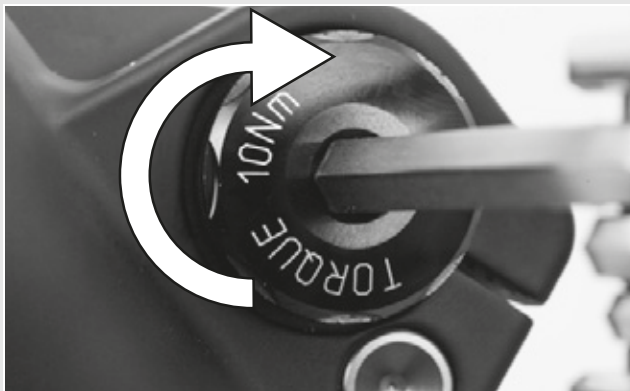
Figura 36: Serraggio del perno inserito
