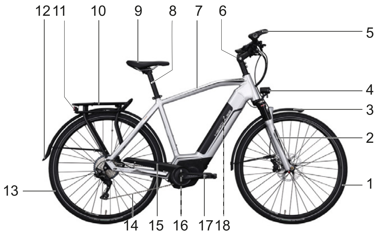
Figura 2: Vista del pedelec da destra, esempio HERCULES Futura Pro 1
