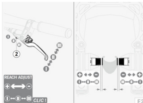
Figura 61: Regolazione dell'ampiezza di presa della leva del freno Magura HS 33
