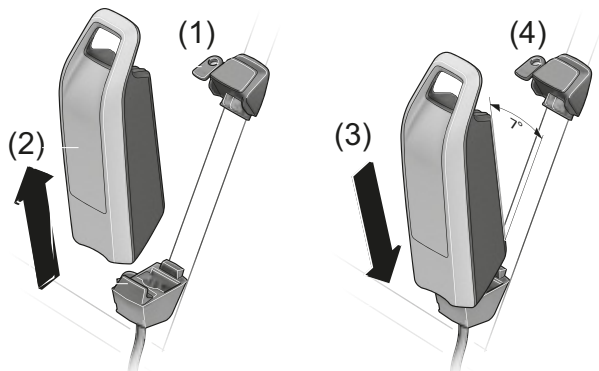
Figura 69: Smontaggio e montaggio della batteria sul tubo trasversale
