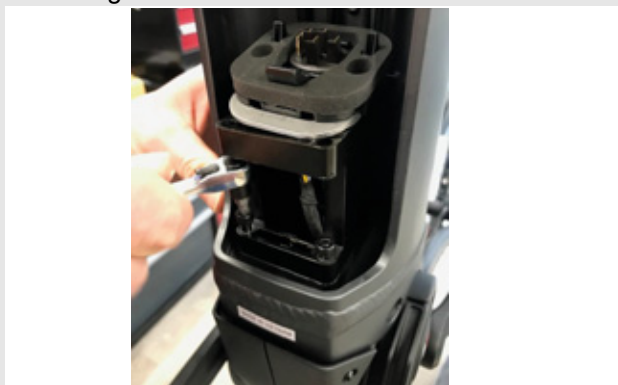
Figura 27: Rimozione delle viti a testa esagonale da 4 mm
