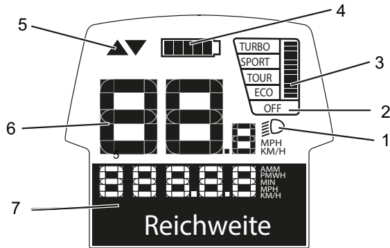
Figura 24: Schema degli indicatori sul display
