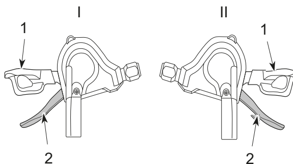
Figura 77: Leva del cambio al rapporto minore (1) e leva del cambio al rapporto maggiore (2) del cambio sinistro (I) e destro (II)
