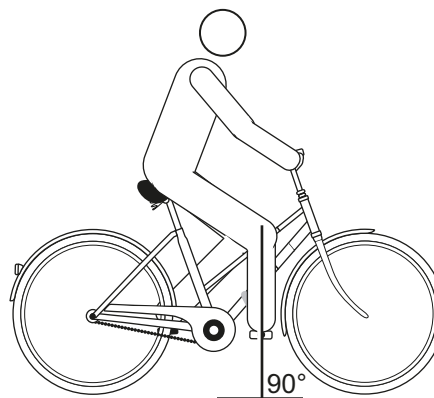
Figura 57: Retta verticale passante per la rotula
