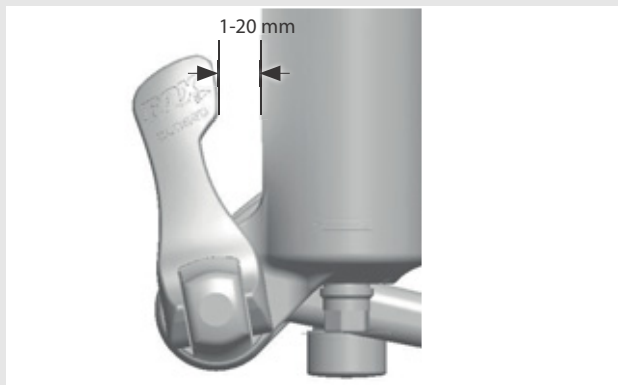
Figura 49: Distanza della leva dal fodero della forcella
