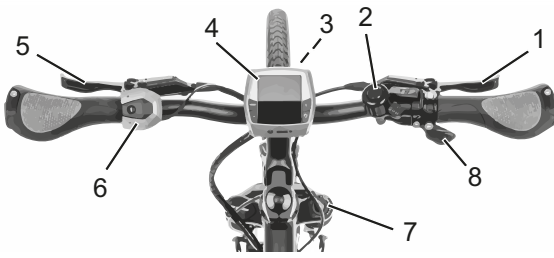
Figura 20: Dettaglio del manubrio visto dalla posizione del ciclista, esempio
