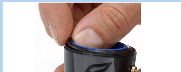
Abbildung 203: Dichtlippenring abziehen
