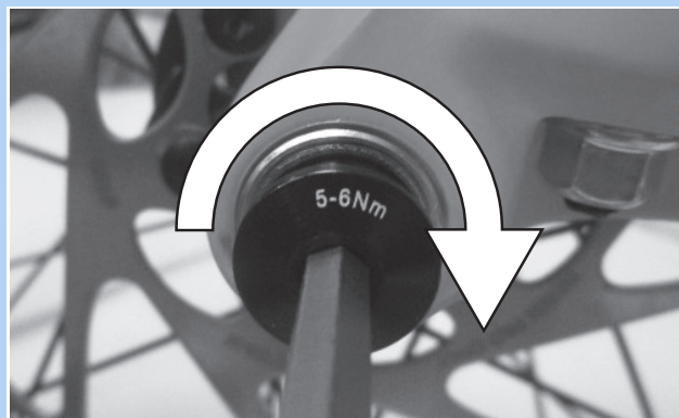
Abbildung 65: Sicherungsschraube anziehen
