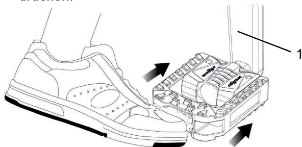
Abbildung 133: Pedal gegen Tretkurbel (1) drücken
