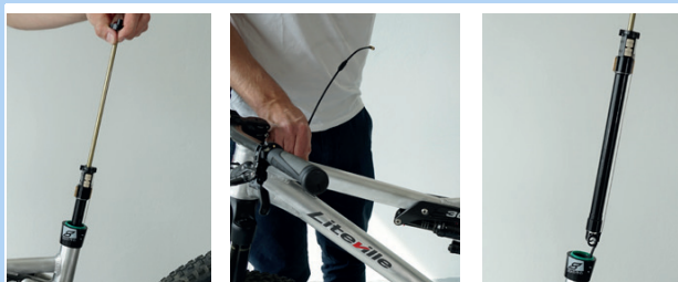
Abbildung 164: Kartusche herausziehen
