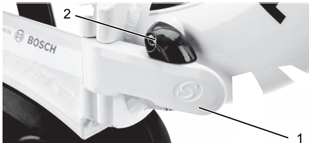
Abbildung 138: Geschlossener Rahmen-Spannhebel (1) und geschlossener Rahmen-Sicherungshebel (2)
