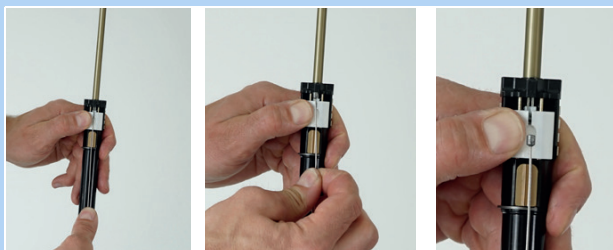
Abbildung 165: Seilzug aushängen
