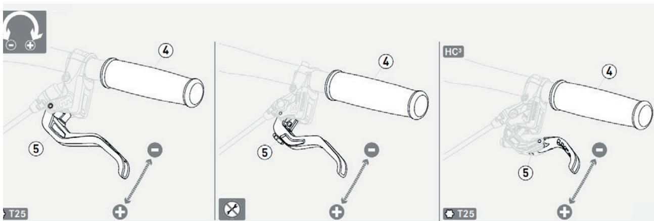
Abbildung 103: Griffweite Bremshebel MAGURA Scheibenbremse einstellen
