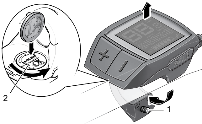
Abbildung 126: Bordcomputer mit Befestigungsschraube (1) und Batteriefachdeckel (2)
